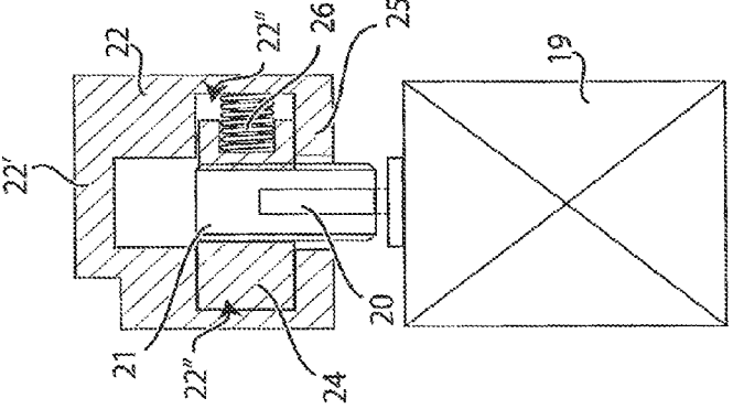
Fig. 11b C-C
