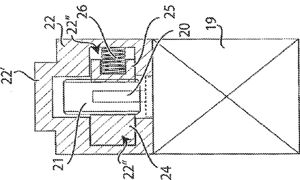
Fig. 10b C-C
