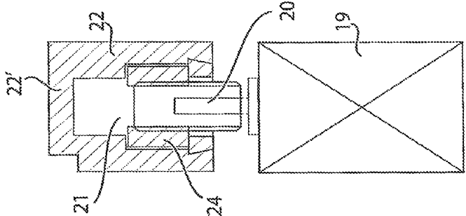
Fig. 11a B-B
