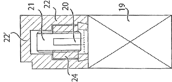
Fig. 10a B-B
