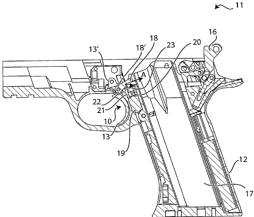
Fig. 5 SECTION A-A
