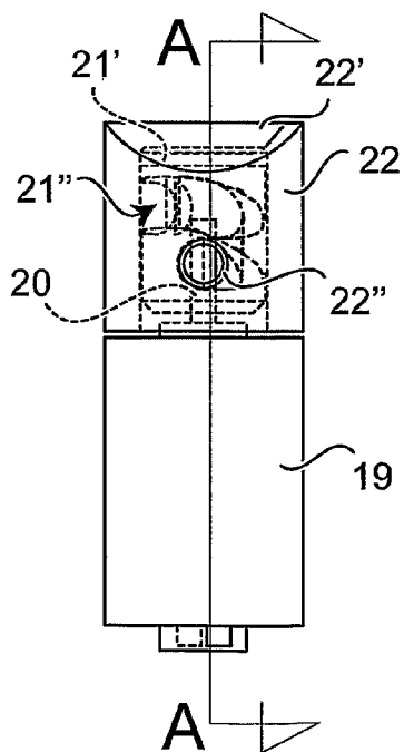
Fig. 12a
