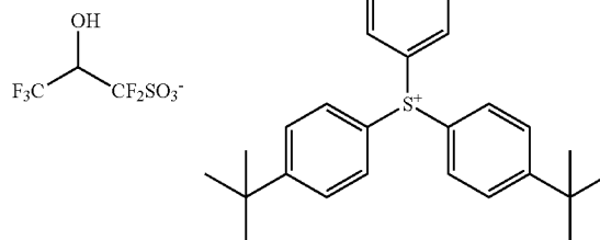
PAG-6
