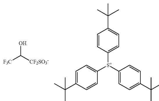
PAG-5
