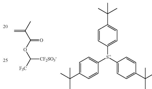
Monomer 5
