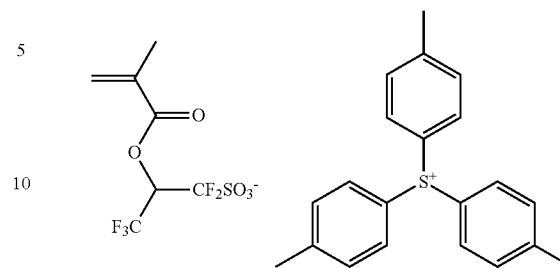
Monomer 5
