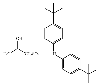
PAG-1
