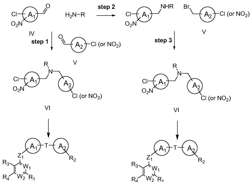
Scheme VI
