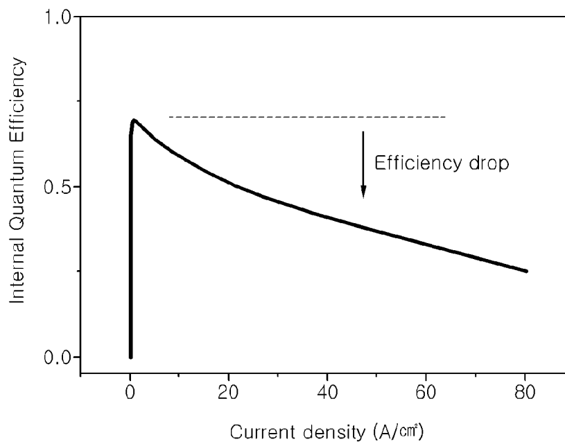
【FIG. 2】 (Related Art)
