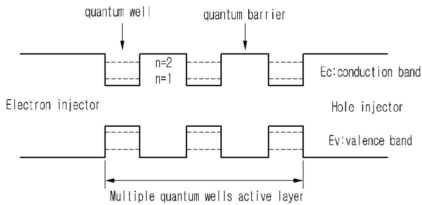
【FIG. 1】 (Related Art)
