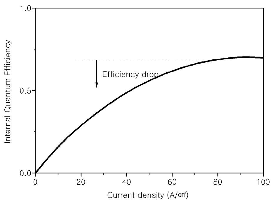
【FIG. 4】 (Related Art)
