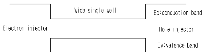
【FIG. 3】 (Related Art)
