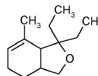
Formula VIIb
