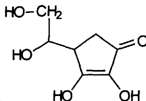
Ascorbinsäure
