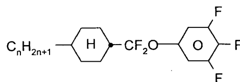
CQU-n-F
