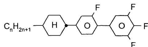
CGU-n-F
