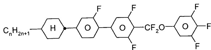
CGUQU-n-F
