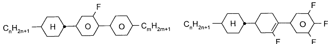
CFU-n-F
