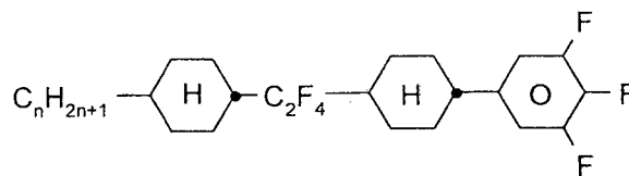
CWCU-n-F
