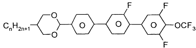
DPGU-n-OT
