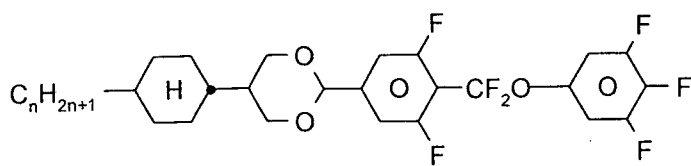
CDUQU-n-F
