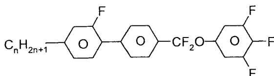
GPQU-n-F
