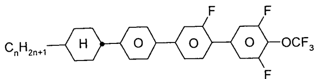
CPGU-n-OT
