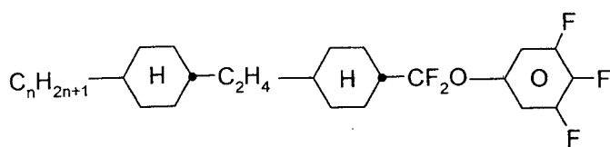
CWCQU-n-F
