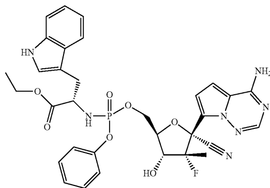
C-3
