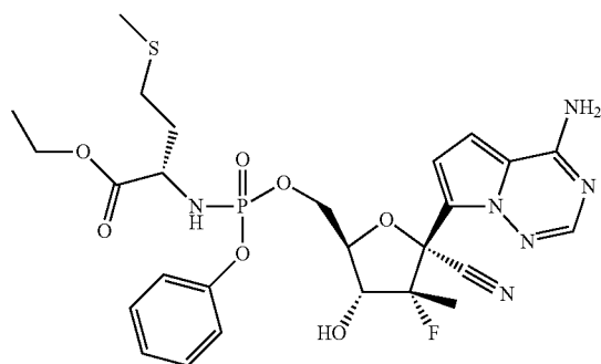
C-2
