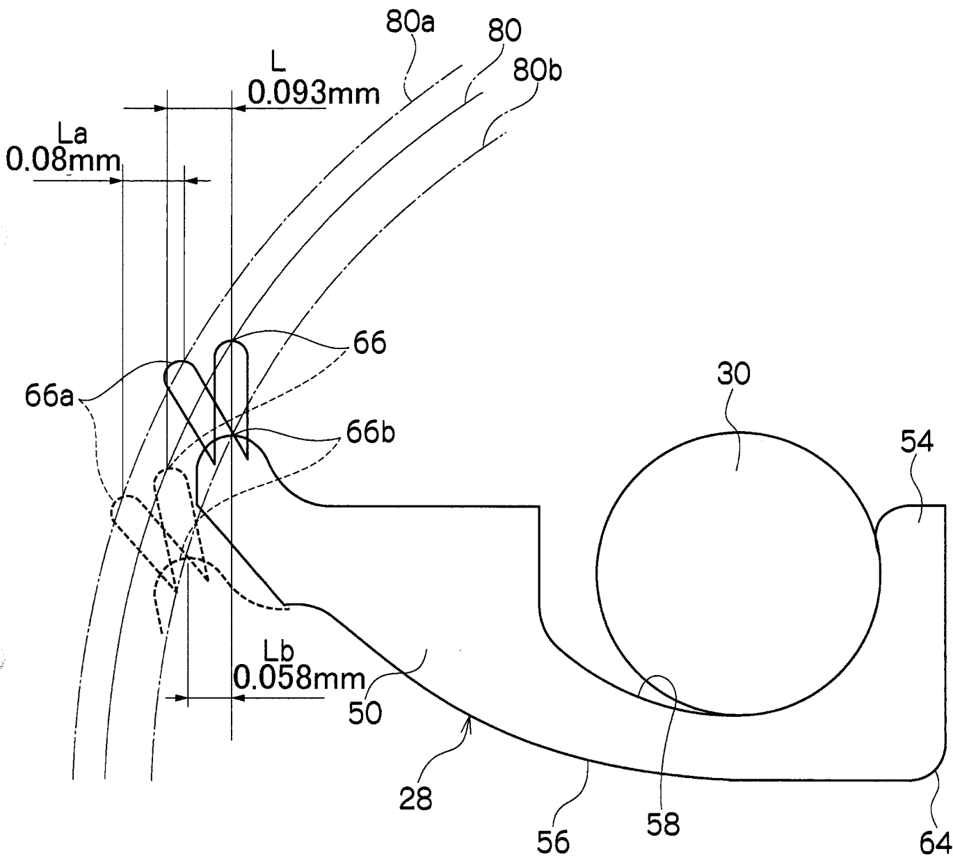
圖 7
