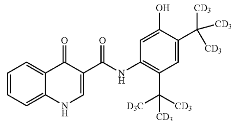
D18-ivacaftor
