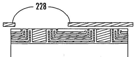
FIG. 4H
