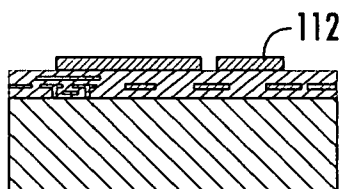
FIG. 3B FRONTSIDE PLATING
