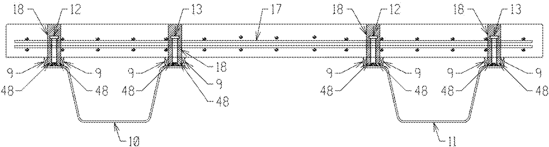
SECTION B-B FIGURE 6G
