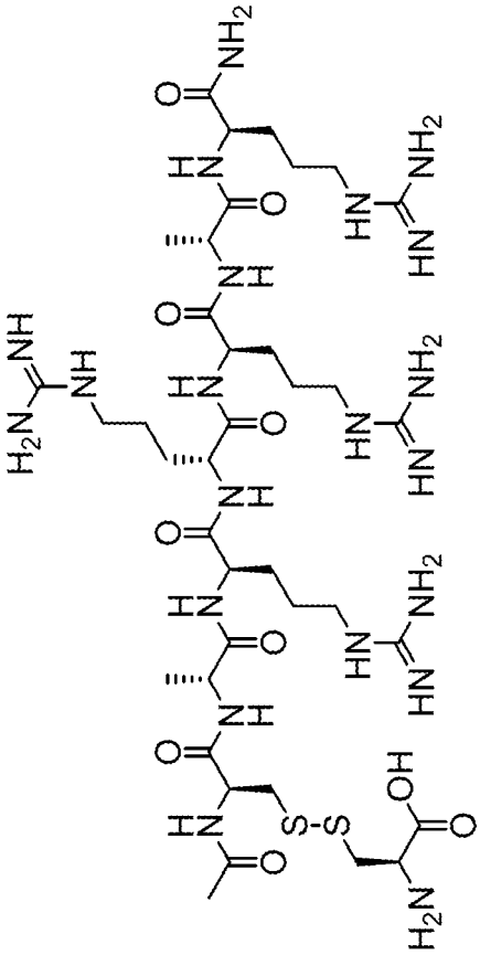
Ac-D-Cys(L-Cys-OH)-D-Ala-D-Arg-D-Arg-D-Arg-D-Ala-D-Arg-NH 2
