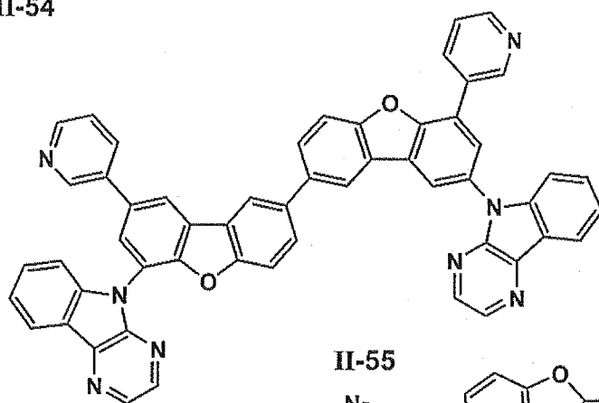
II-54
