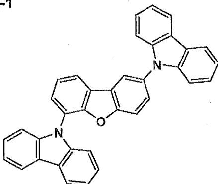
I-1
