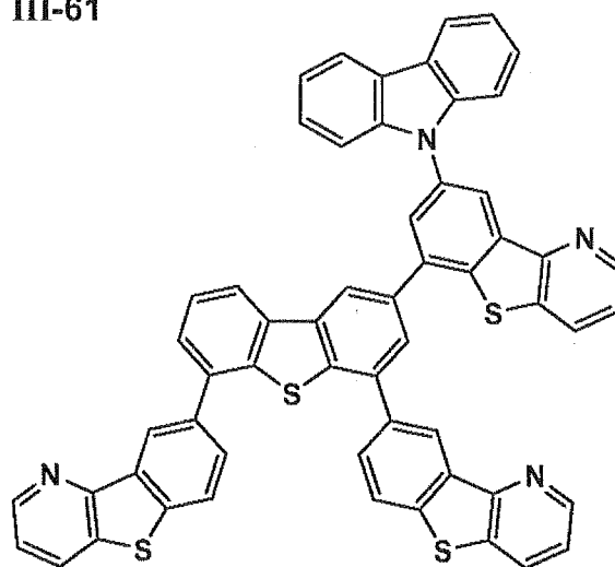
III-61
