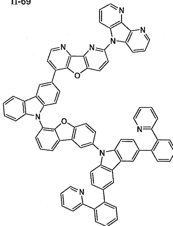
II-69
