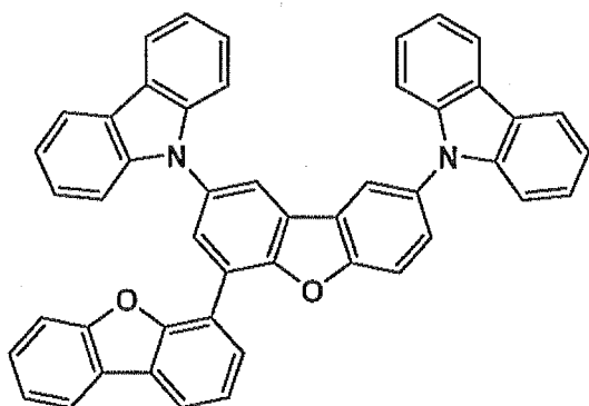
III-60
