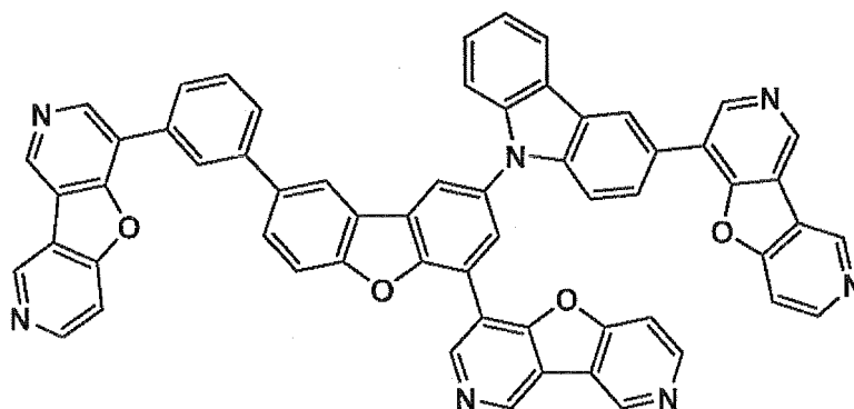
III-63
