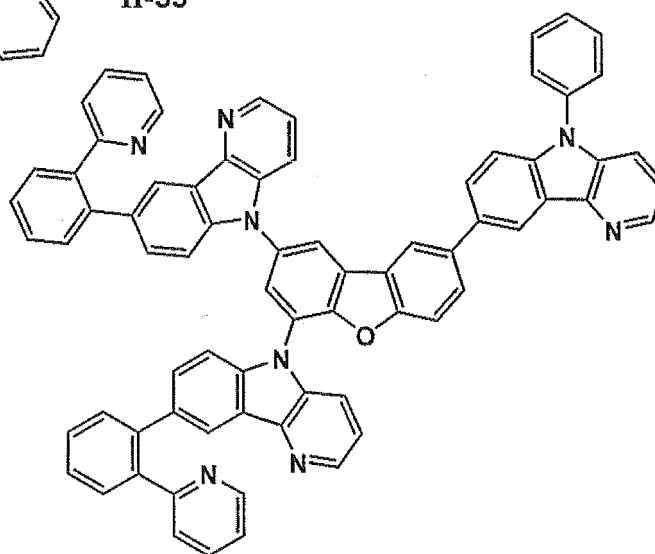
II-35
