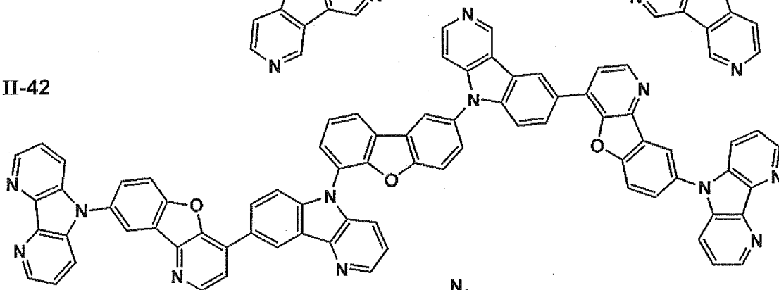
II-43
