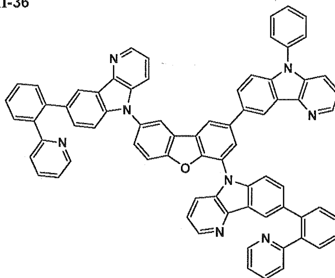
II-36
