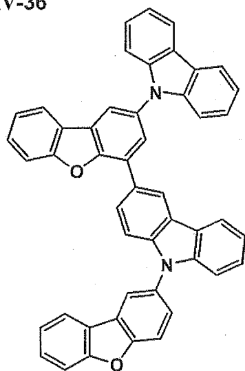
IV-36
