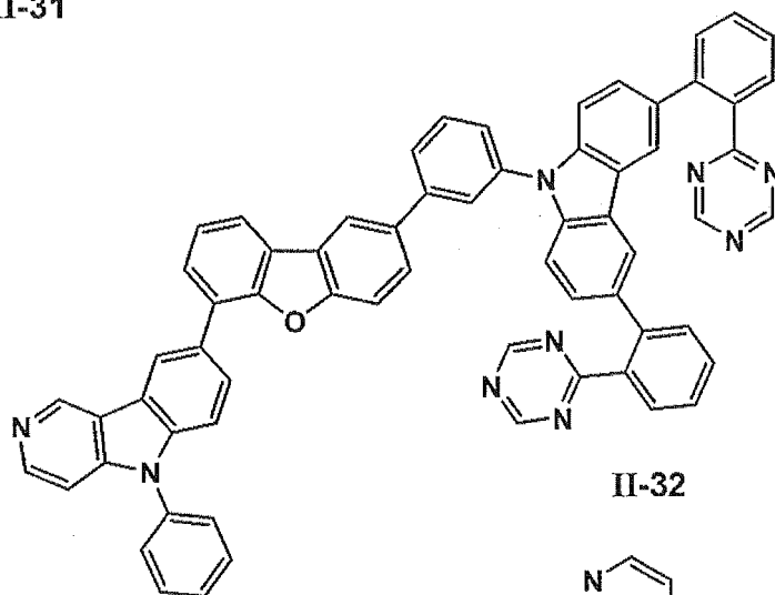
II-31
