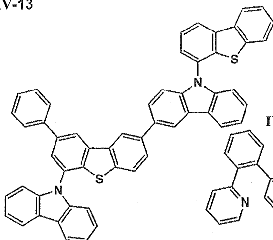
IV-13
