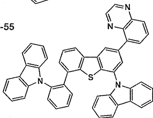
I-57
