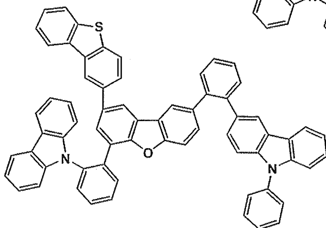
III-44
