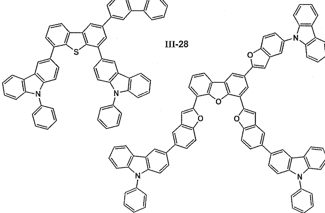
III-27
