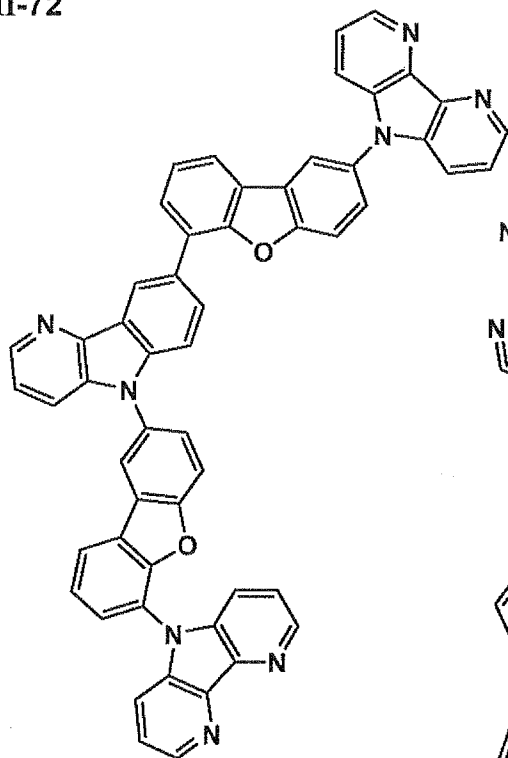
II-72
