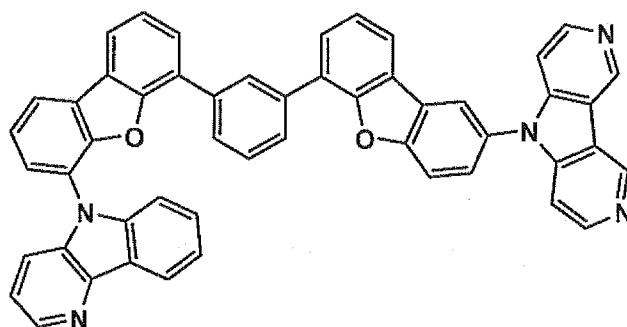
II-74
