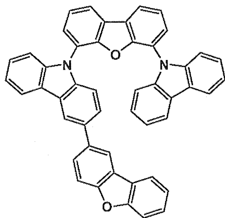
I-63
