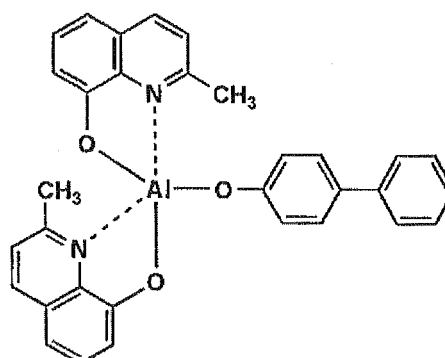
ET-8 (BAIq)
