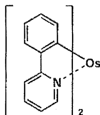
D-22
