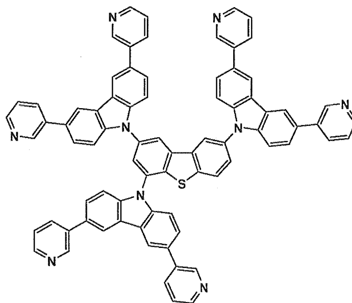
III-14
