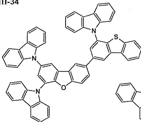
III-34
