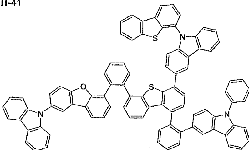
III-41
