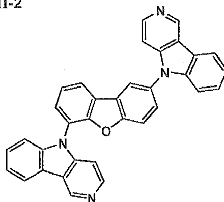
II-2
