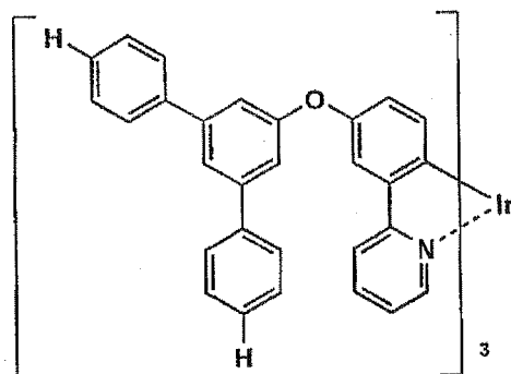
D-13
