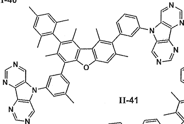
II-40
