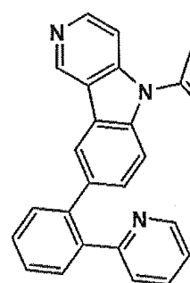
II-20
