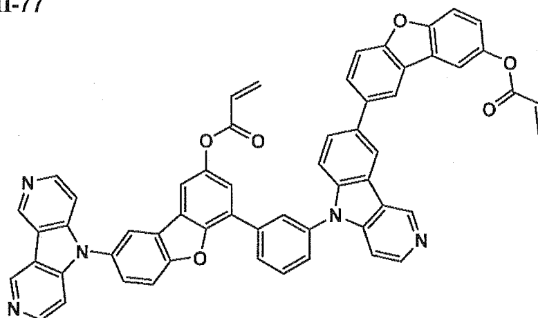
II-77
