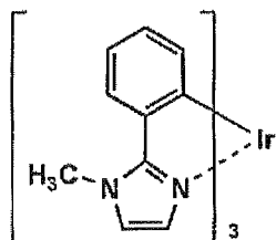
D-24
