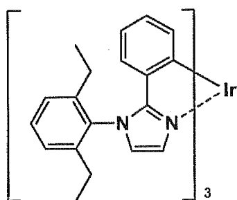
D-48
