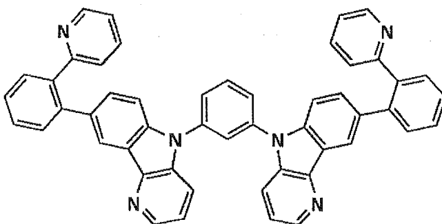
ET-11
