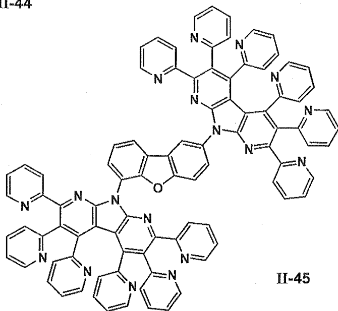
II-44
