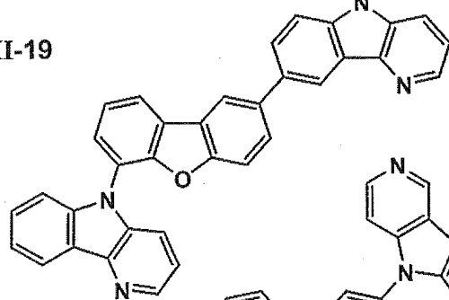
II-20
