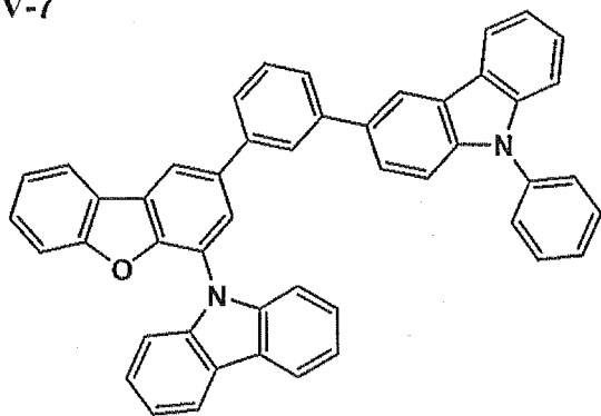
IV-7
