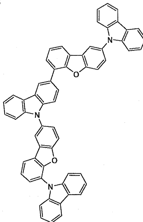
I-66
