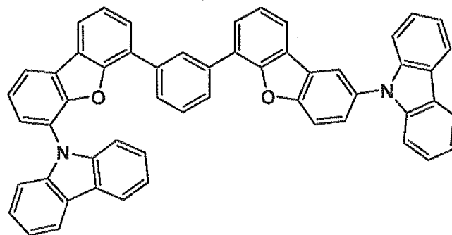
I-68
