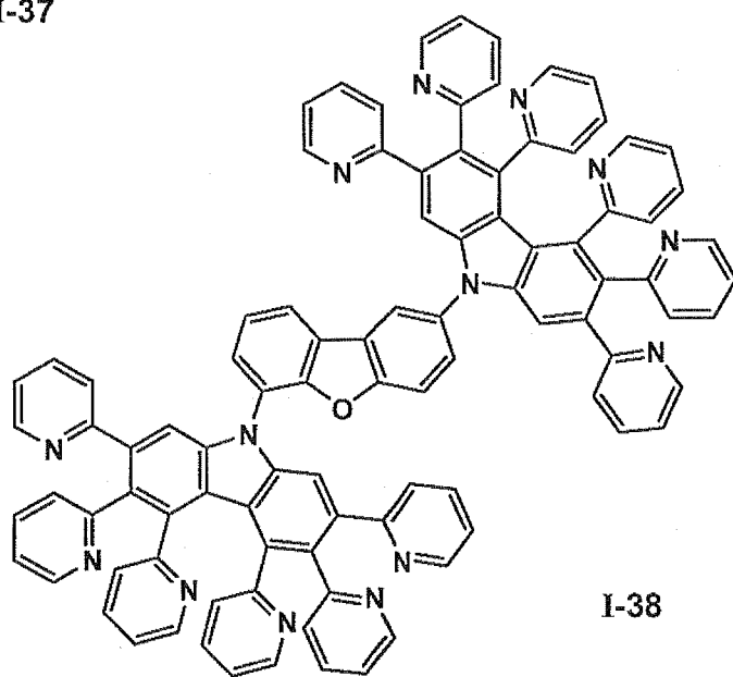
I-37
