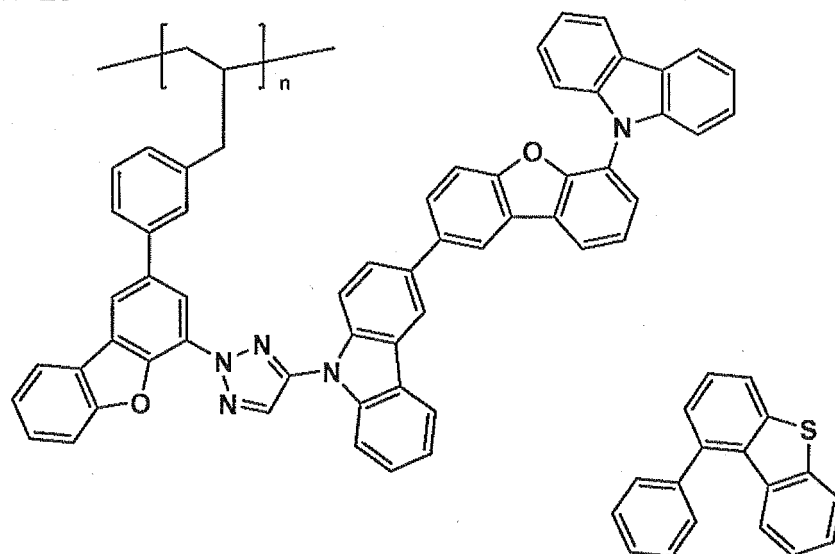
IV-29
