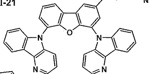
II-21
