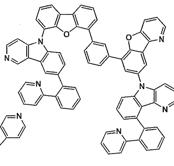
II-47
