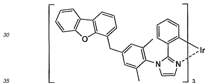
D-44
