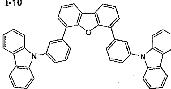
I-10
