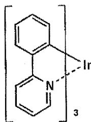
D-1
