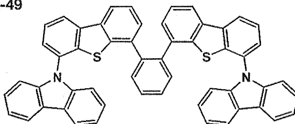
I-49
