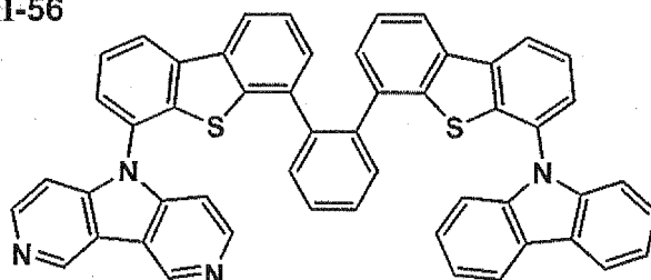
II-56
