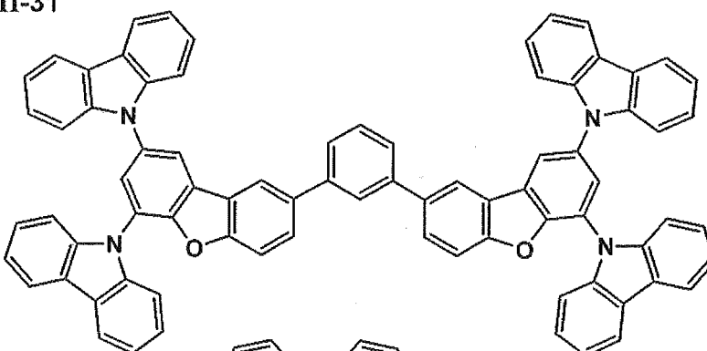
III-32
