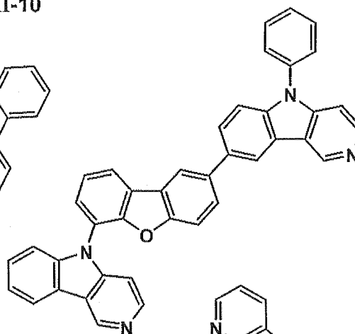
II-12
