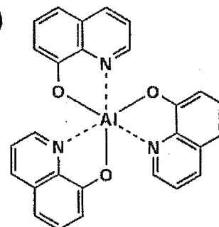
ET-7 (Alq 3 )
