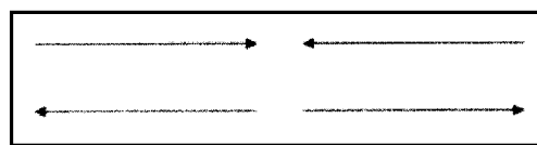
A 1 LAMB WAVE
