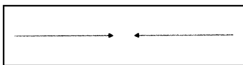
S 0 LAMB WAVE
