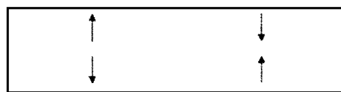
S 1 LAMB WAVE
