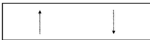
A 0 LAMB WAVE
