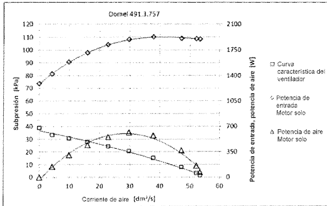
Fig. 4: Datos característicos del aire de una unidad de motor-ventilador con potencia de entrada alta
