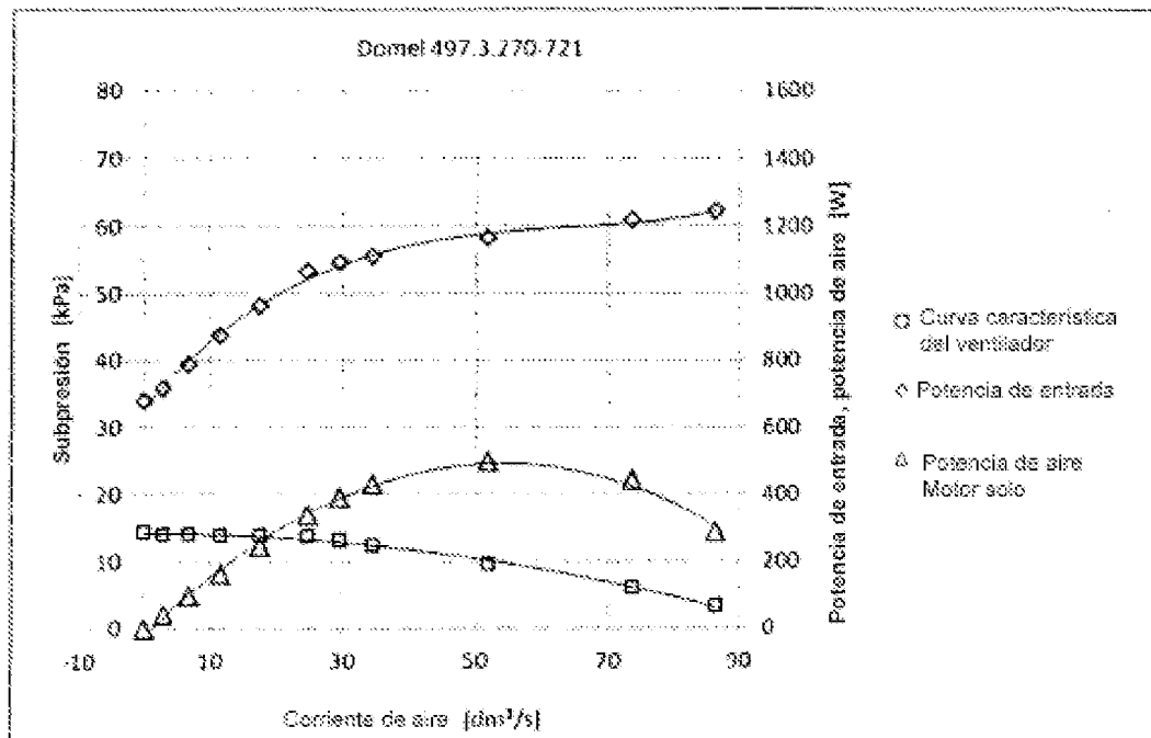
Fig. 5: Datos característicos del aire de una unidad de motor-ventilador para su uso de acuerdo con una realización preferente de la presente invención
