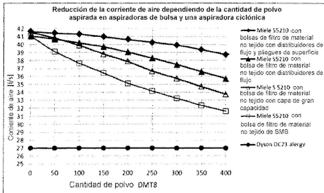
Fig. 3: Reducción de la corriente de aire al aspirar 400 g de polvo de prueba DMT8 de conformidad con la norma EN60312 con una potencia de entrada de 2200 W (Miele S5210) y 1400 W (Dyson DC23 allergy)
