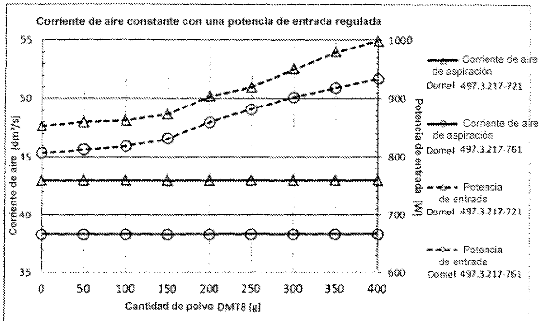
Fig. 6. Aspiradora con potencia de aspiración alta de manera constante y una potencia de entrada inferior a 1000 W
