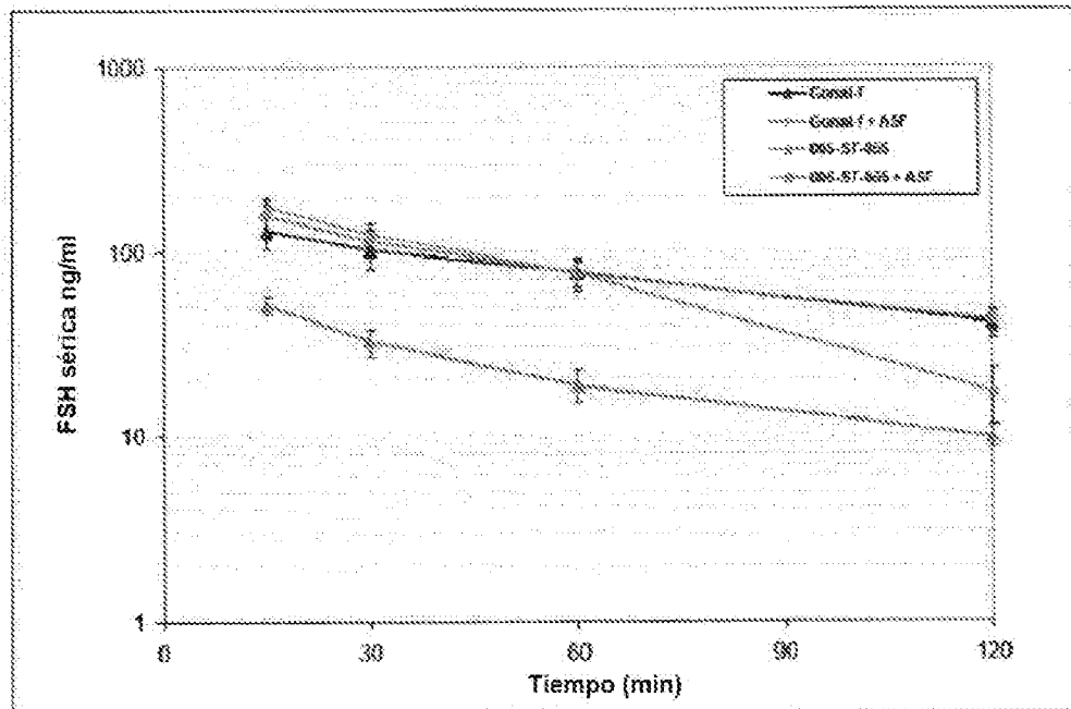
Figura 9. Tasas de eliminación metabólica de muestras de Per.C6-FSH manipuladas con \alpha 2,6 -sialiltransferasa con coadministración de un exceso molar de 7500 veces de asialofetúina para saturar el ASGP-R durante 1-2 h.
