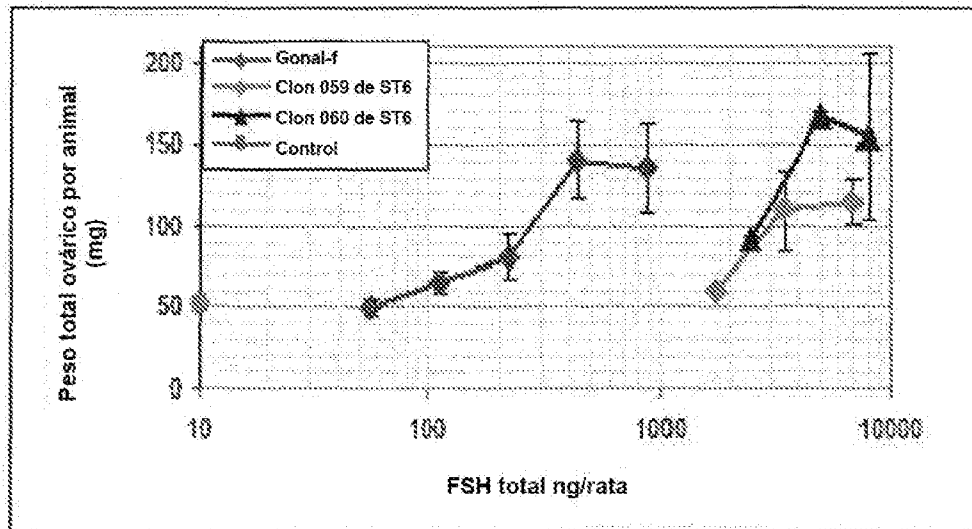
Figura 12. Aumento del peso ovárico según el método de Steelman y Pohley (1953). Se probaron Per.C6-FSHr manipulada con \alpha 2,6 -sialiltransferasa y patrones (Gonal-f FSHr) a diferentes dosis (3 ratas/dosis).
