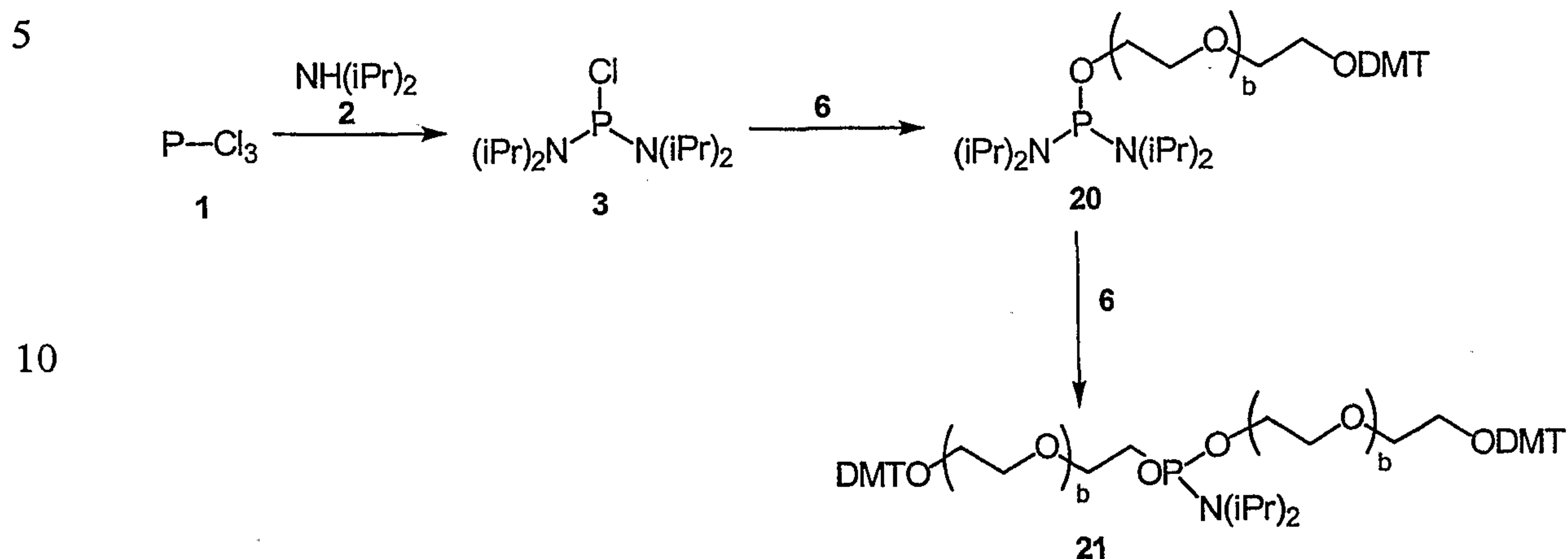
Scheme (IV)
