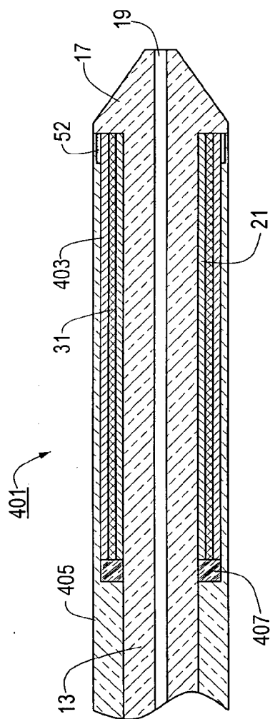
FIG. 16
