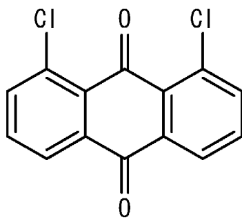
1, 8-ジ クロアントラキノ
