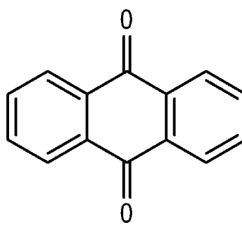
アントラキノ
