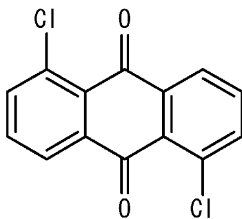
1, 5-ジ クロアントラキノ
