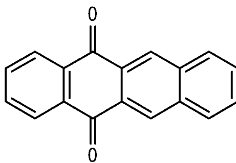
5, 12-ナフトセンキノ
