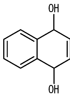
ナフトヒドロキノン
