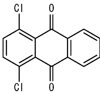
1, 4-ジ クロアントラキノ
