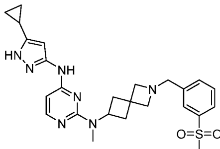
28
