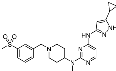
39
