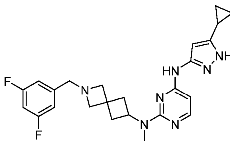
26
