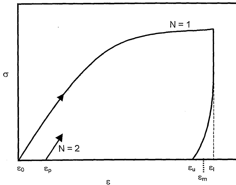
Abb..1: Schematische Darstellung eines dehnungsgeregelten zyklischen thermomechanischen Zug-Dehnungsexperimentes. Die Fixierung der Probe findet bei maximaler Dehnung \epsilon_m bei T_l statt, die Wiederherstellung der Form im entspannten Zustand bei T_h .
