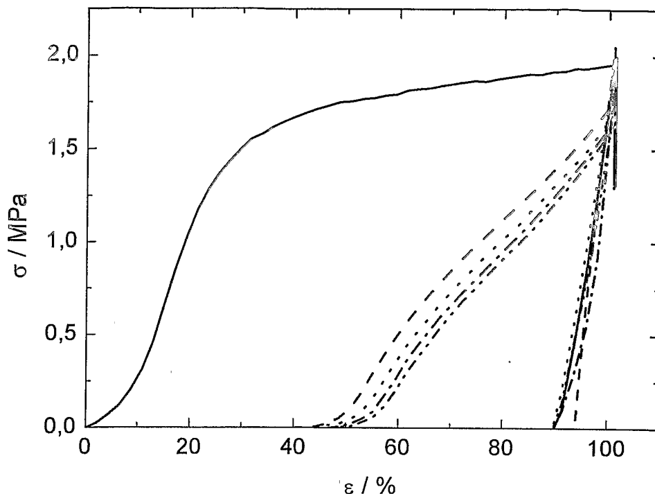
Abb. 6: Darstellung eines dehnungsgeregelten, zyklischen, thermomechanischen Zug-Dehnungsexperimentes am Beispiel der extrudierten Polymermischung PDA(50)/PCA(68)[30/27] mit T_h = 50 \text{ }^\circ\text{C} , T_l = 0 \text{ }^\circ\text{C} und \epsilon_m = 100 \text{ } \% .
