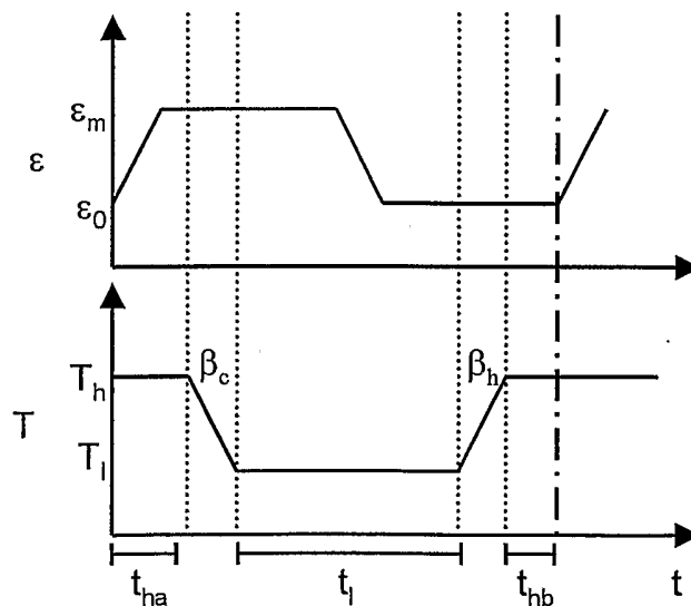
Abb.2: Schematische Darstellung des Prinzips des dehnungsgeregelten thermomechanischen Zyklus. Die Änderung der Temperatur von T_h zu T_l bzw. T_l zu T_h ist mit einer gepunkteten Linie (.....) angedeutet. Die letzte vertikale Linie (- - -) kennzeichnet das Ende des ersten Zyklus.
