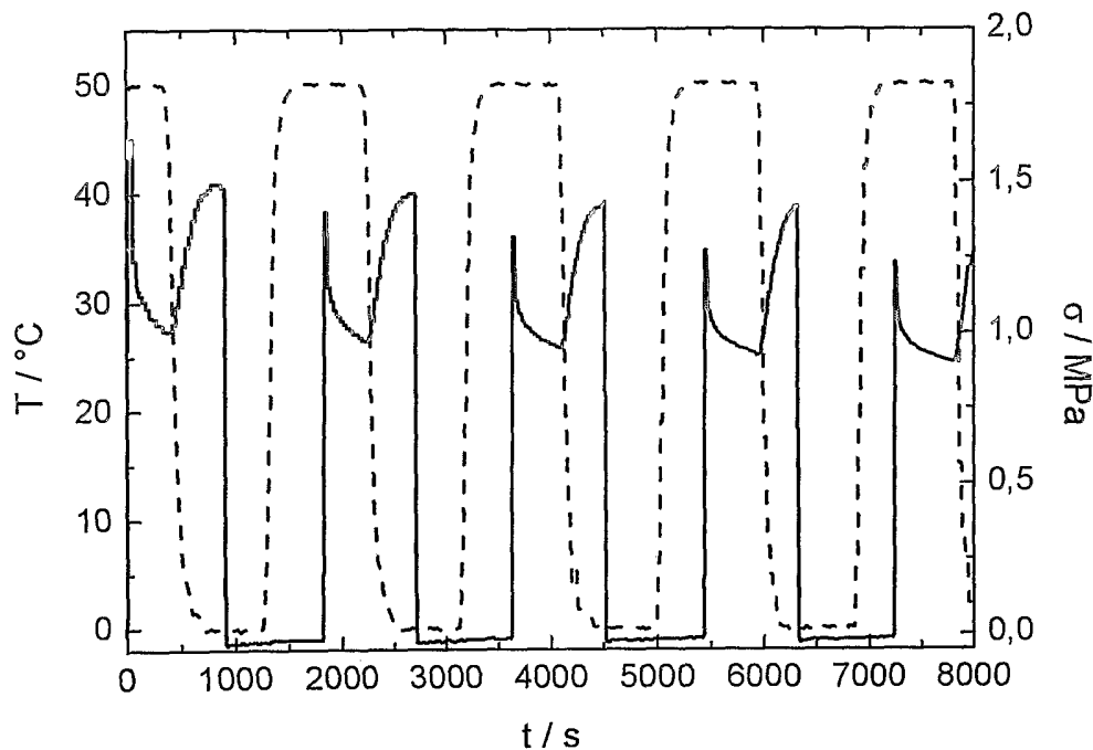
Abb. 4: Temperatur T (---) und Spannung \sigma (-) in Abhängigkeit von der Zeit während eines dehnungsgeregelten zyklischen thermomechanischen Zyklus am Beispiel der Polymermischung PDA(50)/PCA(47)[22/28].
