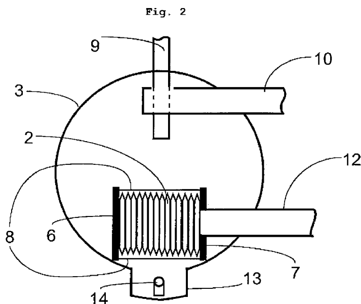
Anordnung der Wärmeübertragungsplatten
