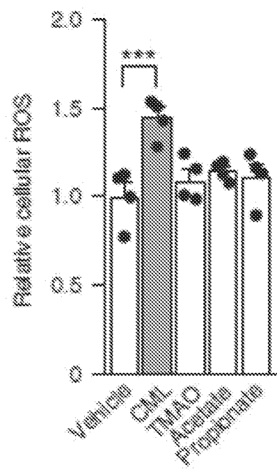
ROS
