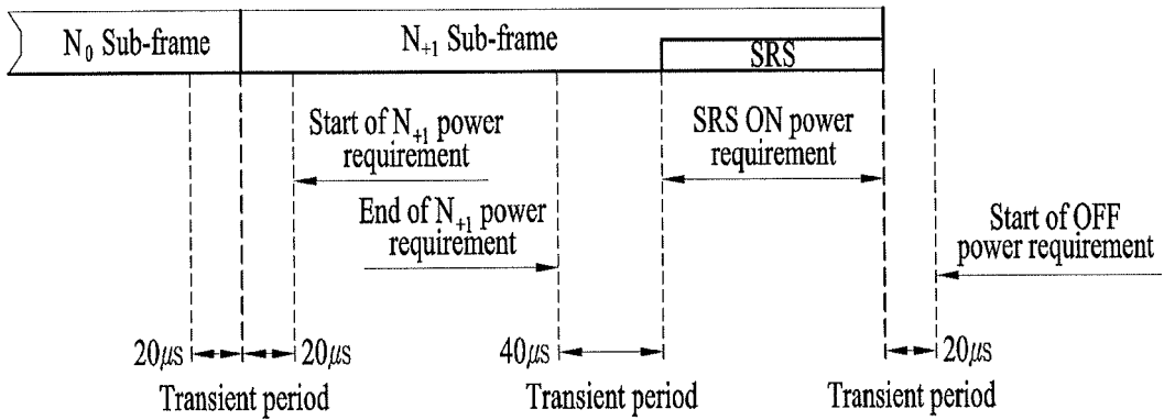
FIG. 19E
