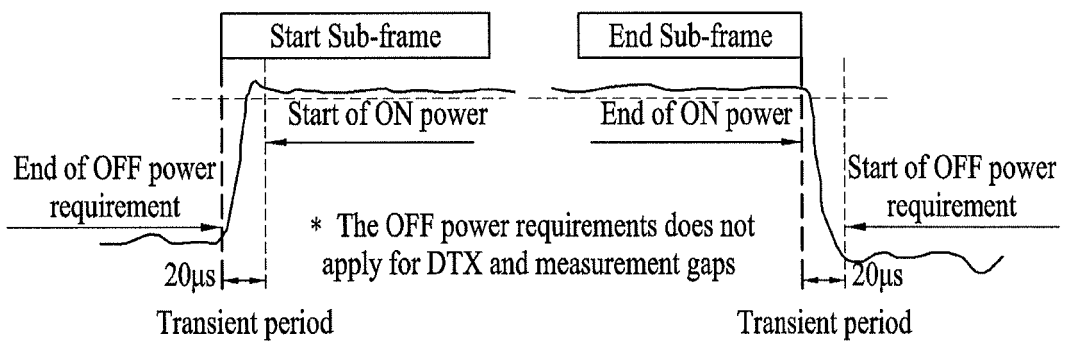
FIG. 19A
