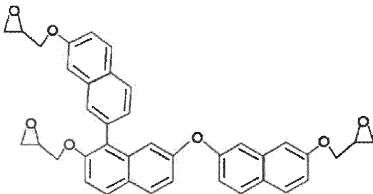
[Chem 25]
