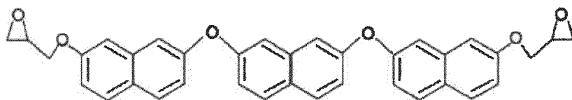
[Chem 25]
