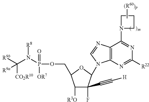
Formula IVb'
