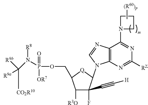
Formula IVb'
