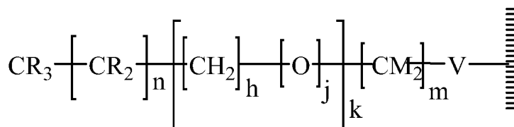
Formel II:
