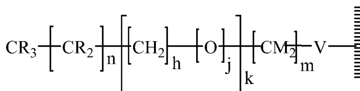
Formula II:
