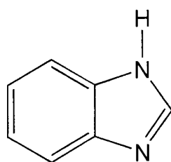
Benzimidazole
