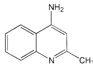
4-Amino quinaldine
