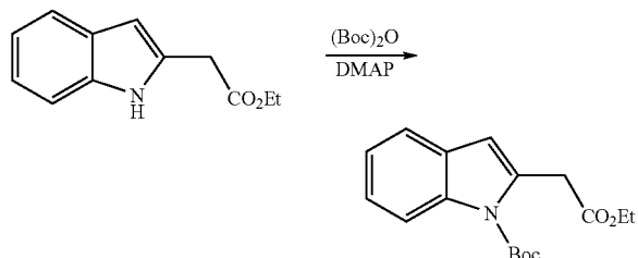
tert-Butyl 2-((ethoxycarbonyl)methyl)-1H-indole-1-carboxylate
