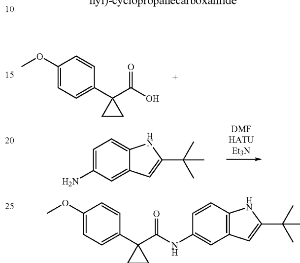
N-(2-tert-Butyl-1H-indol-5-yl)-1-(4-methoxyphenyl)-cyclopropanecarboxamide
