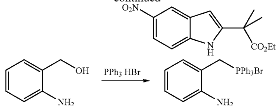
Triphenyl(2-aminobenzyl)phosphonium bromide
