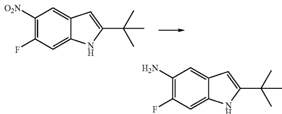
2-tert-Butyl-6-fluoro-1H-indol-5-amine
