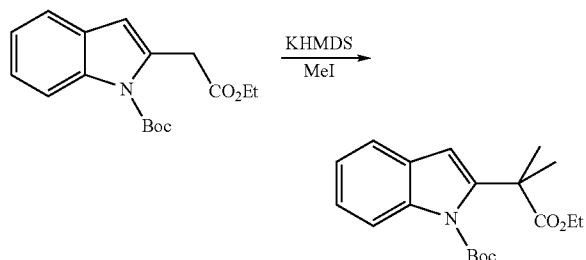
tert-Butyl 2-(2-(ethoxycarbonyl)propan-2-yl)-1H-indole-1-carboxylate
