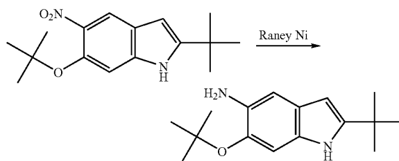
6-tert-Butoxy-2-tert-butyl-1H-indol-5-amine
