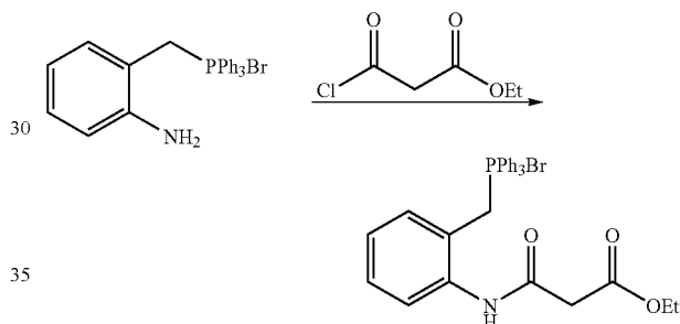
Triphenyl((ethyl(2-carbamoyl)acetate)-2-benzyl)phosphonium bromide
