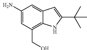
(5-Amino-2-tert-butyl-1H-indol-7-yl)methanol
