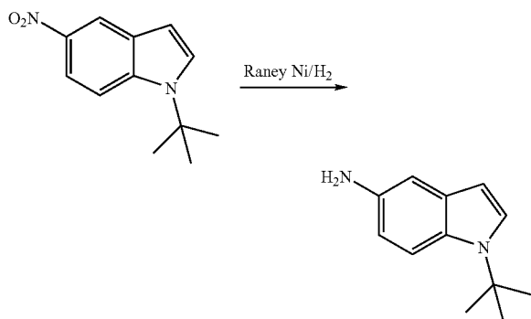
1-tert-Butyl-1H-indol-5-amine
