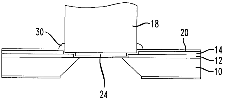
FIG. 3F
