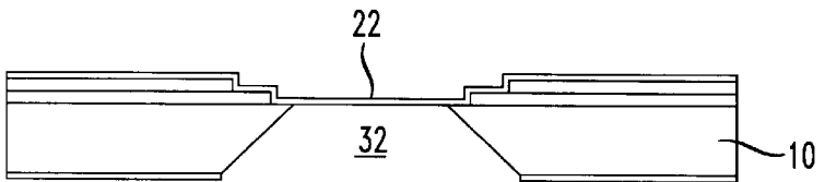
FIG. 3E
