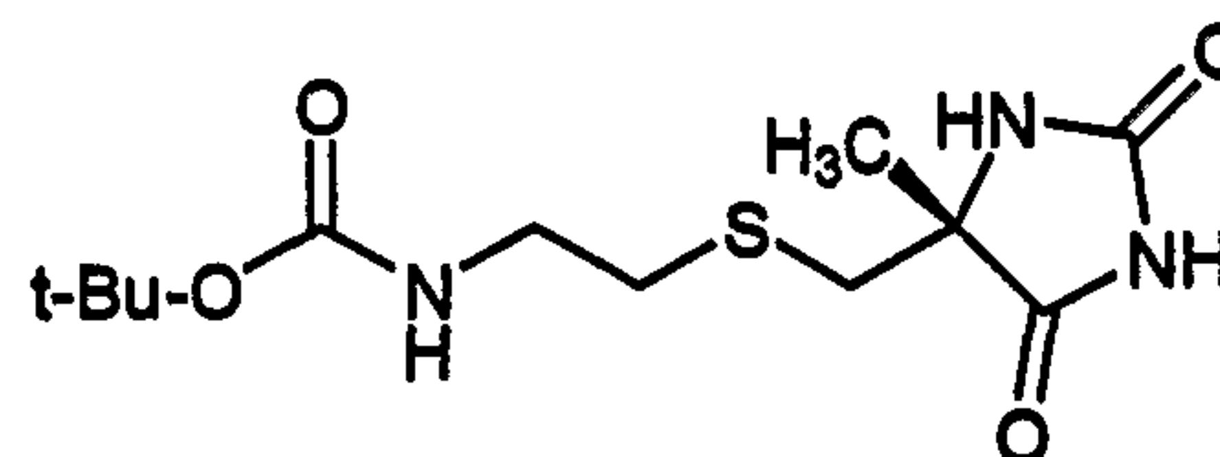
R enantiomer
