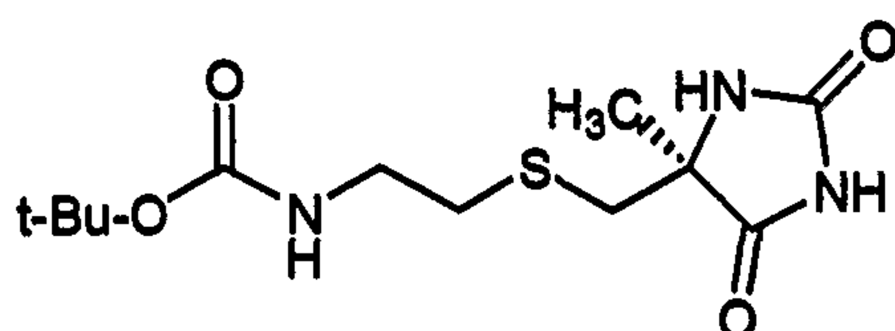
S enantiomer
