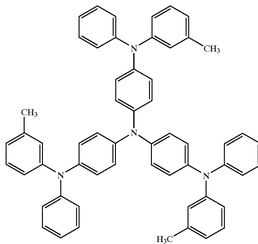
m-MTDATA (T g = 75° C.)
