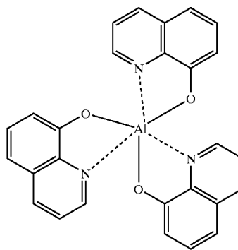
Almq 3
