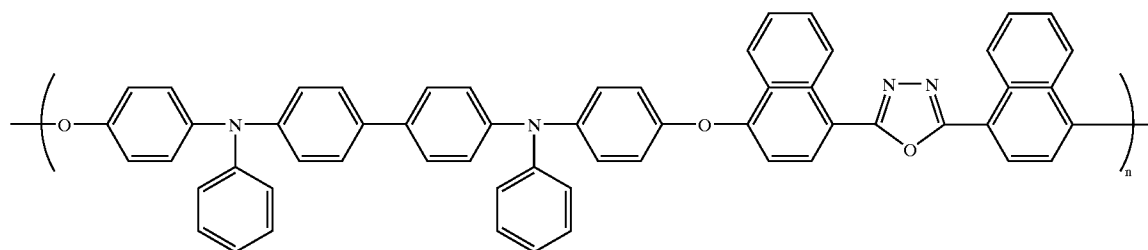
PTPDOXD
