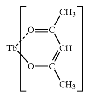
Tb(acac) 3
