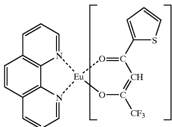
Eu(TTFA) 3 Phen
