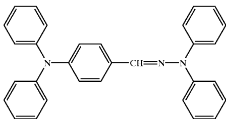
DPH
