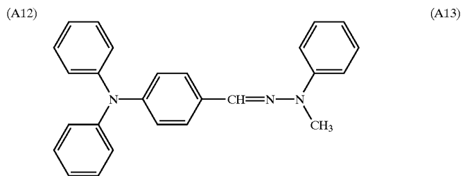
PTPAEK
