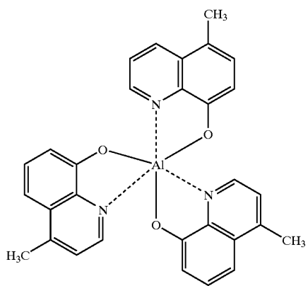
Almq 3
