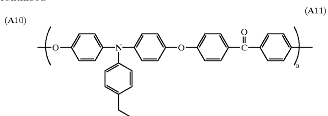
PTPAEK
