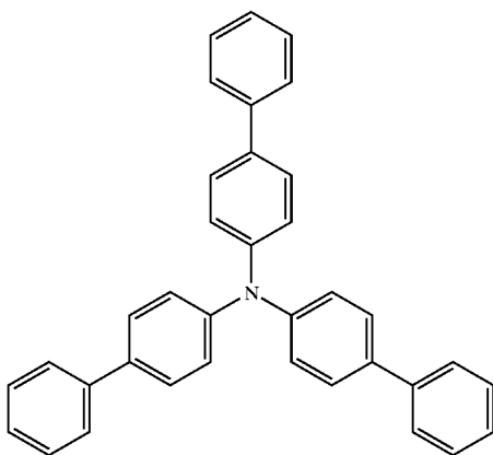
ECMH
