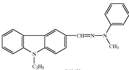
ECMH
