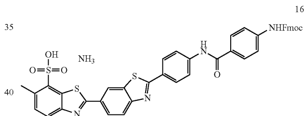
2'-(4-(4-(((9H-fluoren-9-yl)methoxy)carbonyl)amino)benzamido)phenyl)-6-methyl-[2,6'-bibenzo[d]thiazole]-7-sulfonic acid (16)
