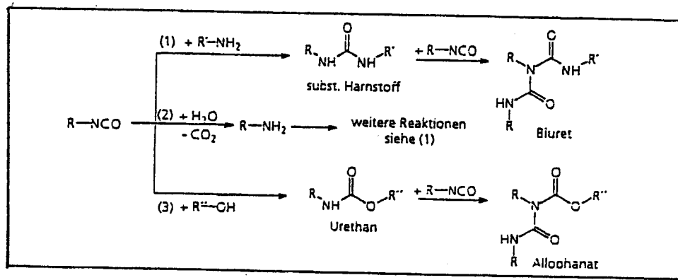
Fig. 1 : Wichtige Reaktionen von Isocyanaten
