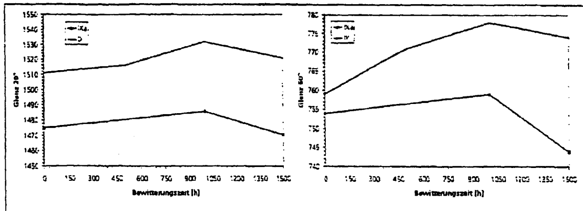
Fig. 11: Zeitabhängige Veränderung des Glanzes der Schichten IV und V bei Bewitterung im QUV-B Test (Glanzwerte bei 20° und 60°)
