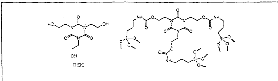
Fig. 10: Monomerer Triol und mögliches Produkt der Härungsreaktion von System IV
