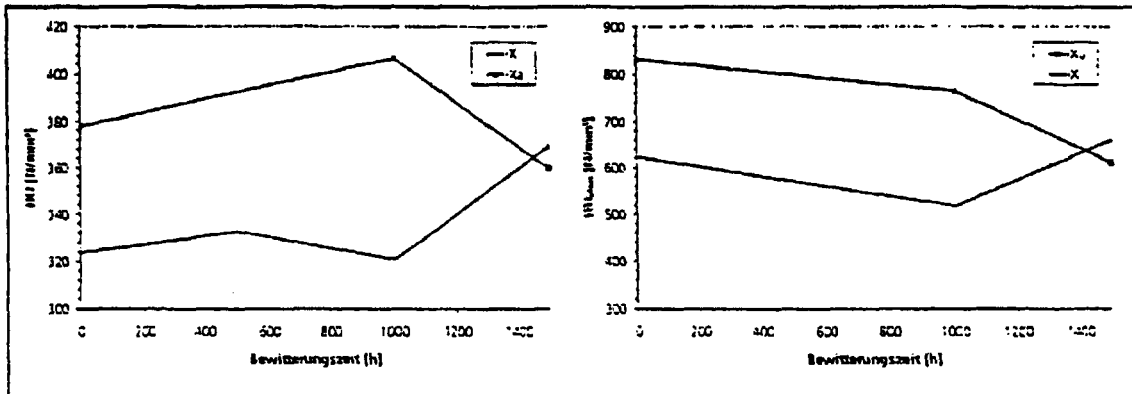
Fig. 13: Zeitabhängige Änderung der Universalhärte und der plastischen Universalhärte der Systeme IV und V nach Belastung im QUV-B Test
