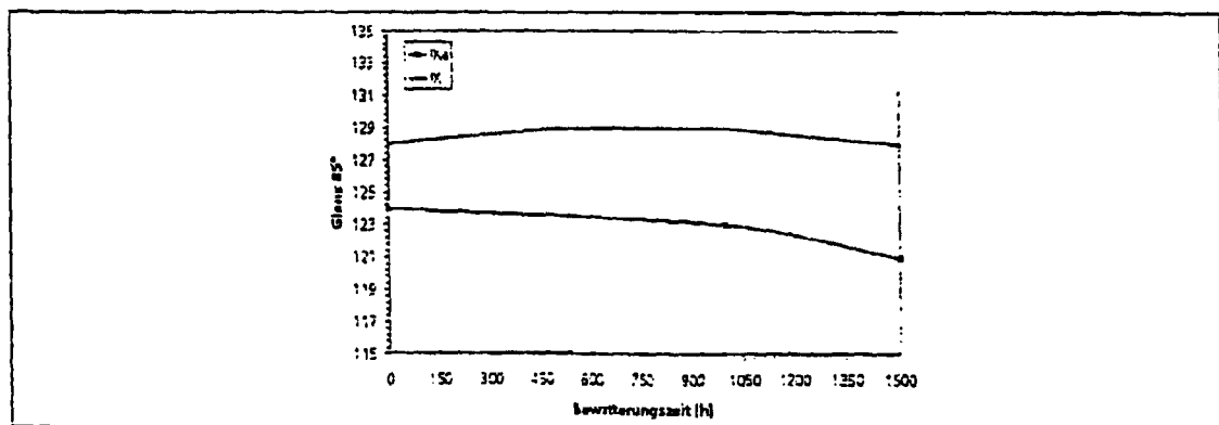
Fig. 12: Zeitabhängige Veränderung des Glanzes der Schichten IV und V bei Bewitterung im QUV-B Test (Glanzwerte bei 85°)
