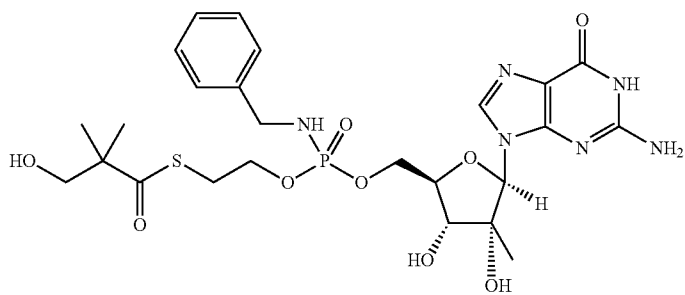
IDX-184
