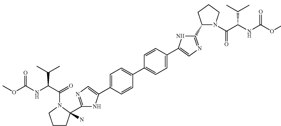
BMS-790052 (daclatasvir)
