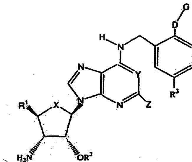
Formule I
