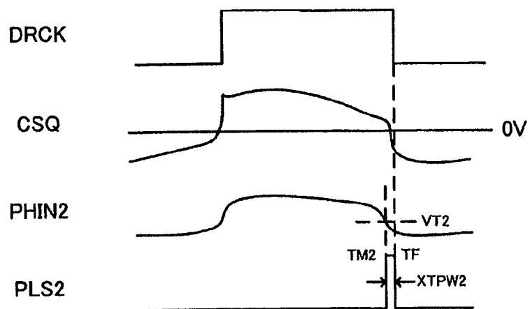
FIG. 14A LOW LOAD
