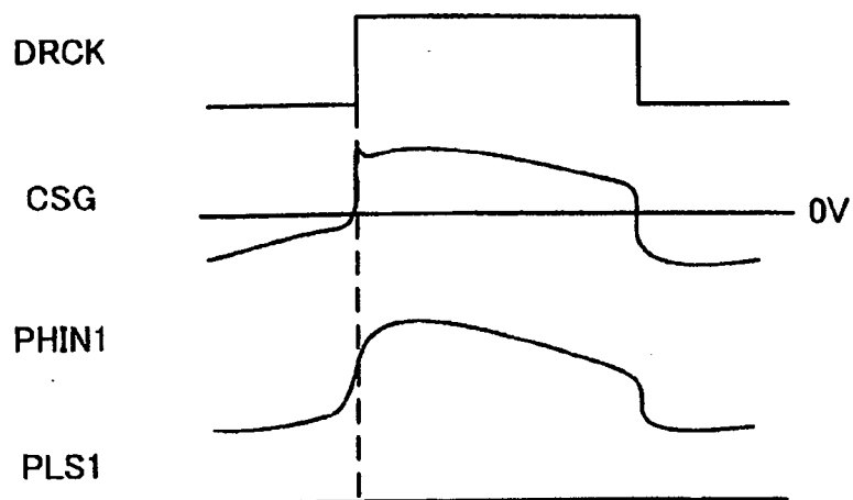
FIG. 9A LOW LOAD
