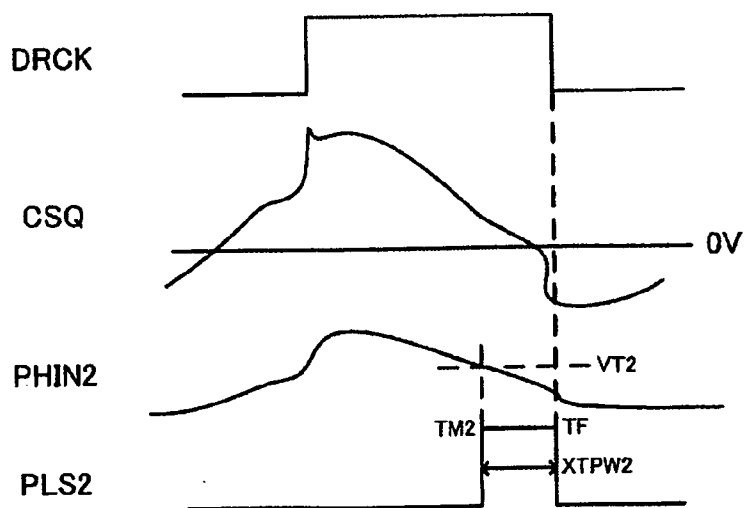
FIG. 14C HIGH LOAD
