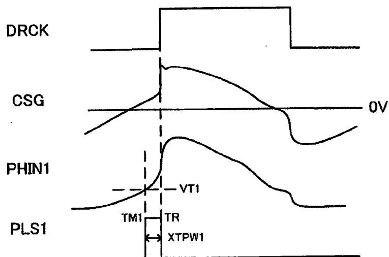
FIG. 9C HIGH LOAD
