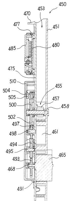
A-A断面図
