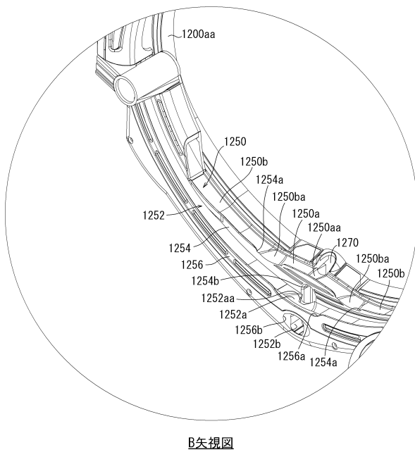
B矢視図
