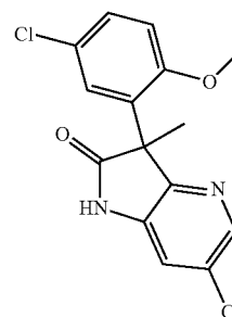
Example 31: 6-chloro-3-(6-chloro-3-methoxypyridin-2-yl)-3-methylindolin-2-one
