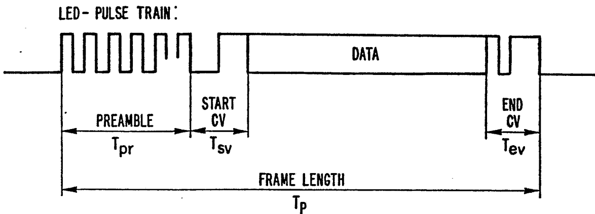
FIG. 3 FRAME FORMAT
