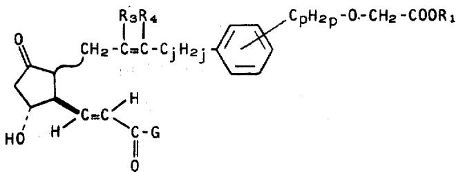
XVII
