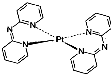
Verbindung 4 (Vergleichsbeispiel)
