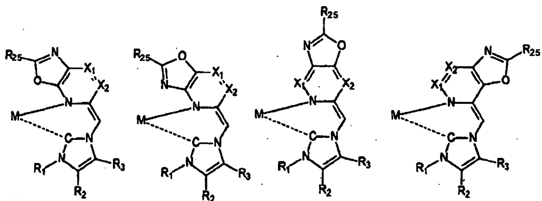
Formel 15
