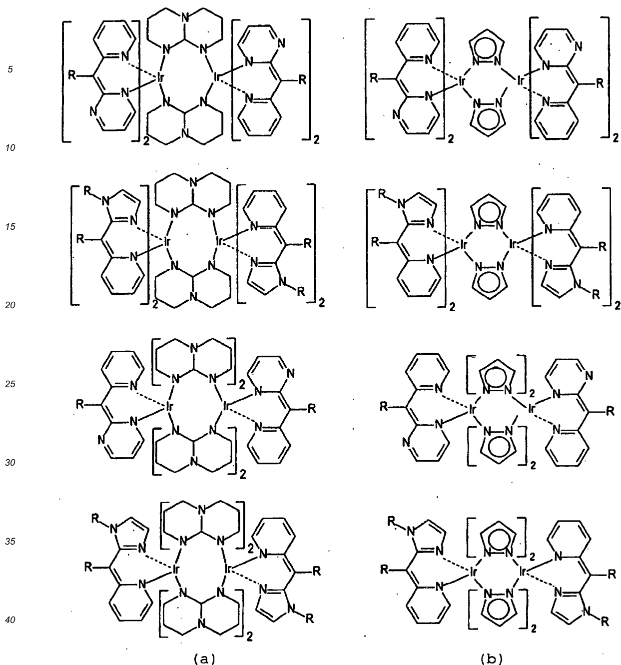
Formel 27 (Vergleichsbeispiele)
