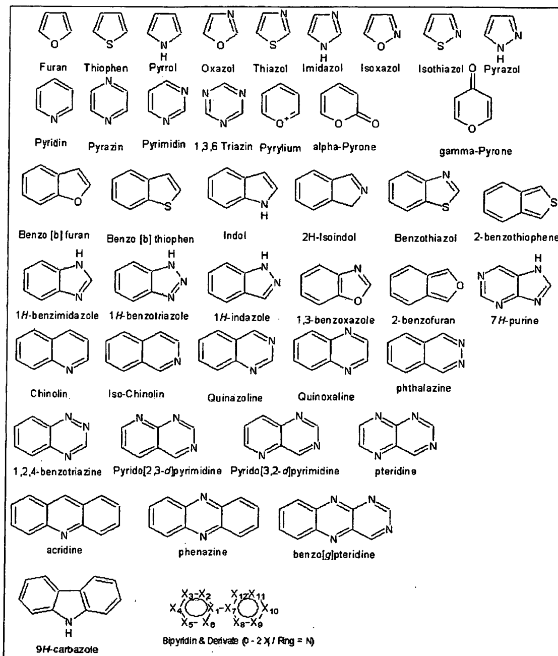
Formel 4
