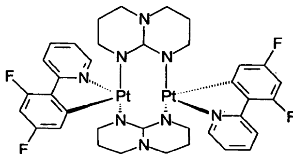
Verbindung 9 (Vergleichsbeispiel)
