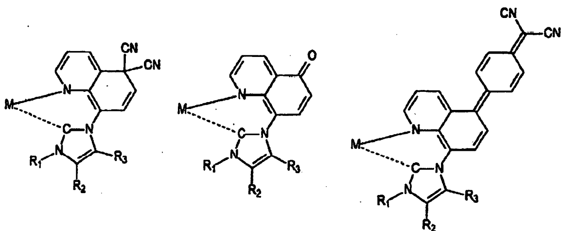
Formel 15
