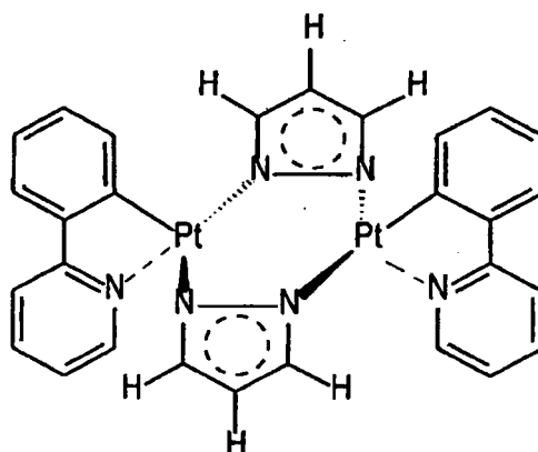
Verbindung 6 (Vergleichsbeispiel)
