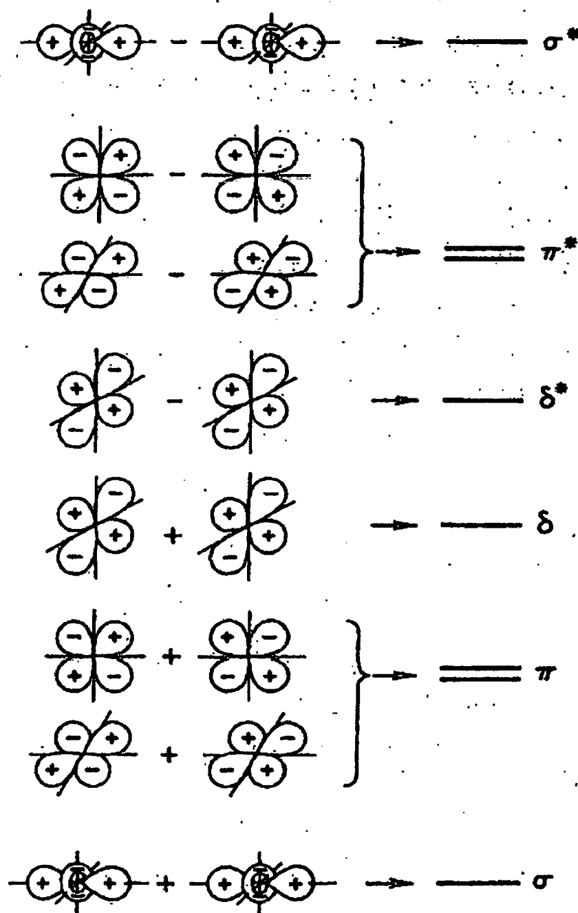
Schema 1
