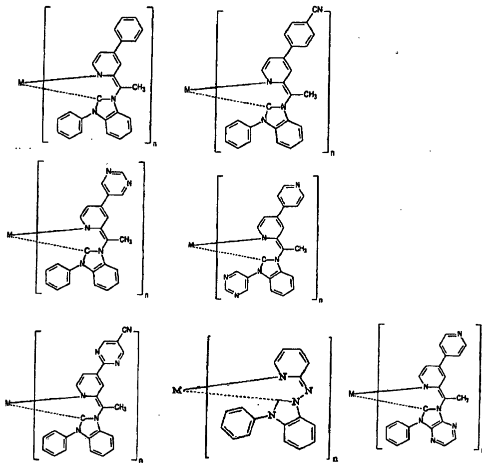
Formel 24
