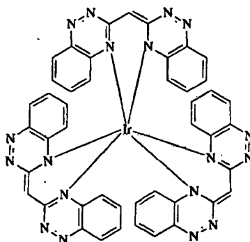
Formel 30 (Vergleichsbeispiel)
