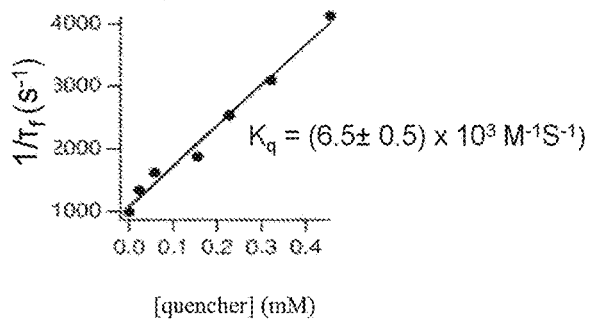
Alkoxy crylene
