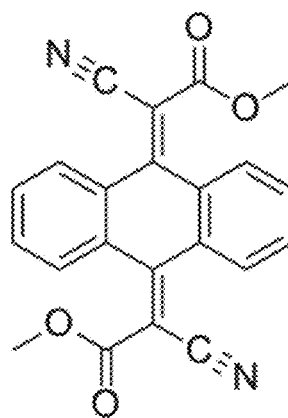
Formula IIei
