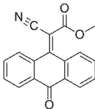
Formula IIci
