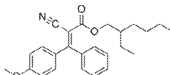
Alkoxy crylene
