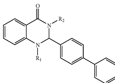
Amide/Amine Substitutions
