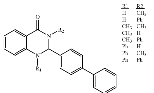
Amide/Amine Substitutions
