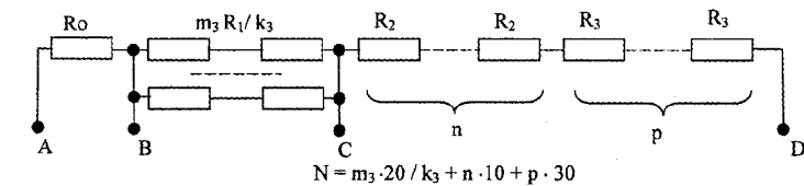
Fig. 5. Exemplu de realizare. A doua etapă – acordarea celui de-al doilea braț al divizorului de tensiune
