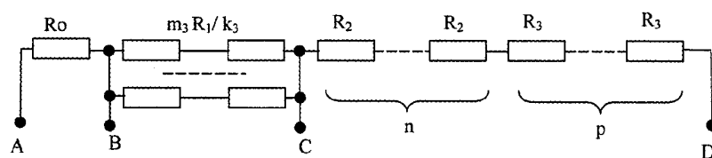
Fig. 2. A doua etapă. Acordarea celui de-al doilea braț (al treptelor a doua și a treia) al divizorului de tensiune
