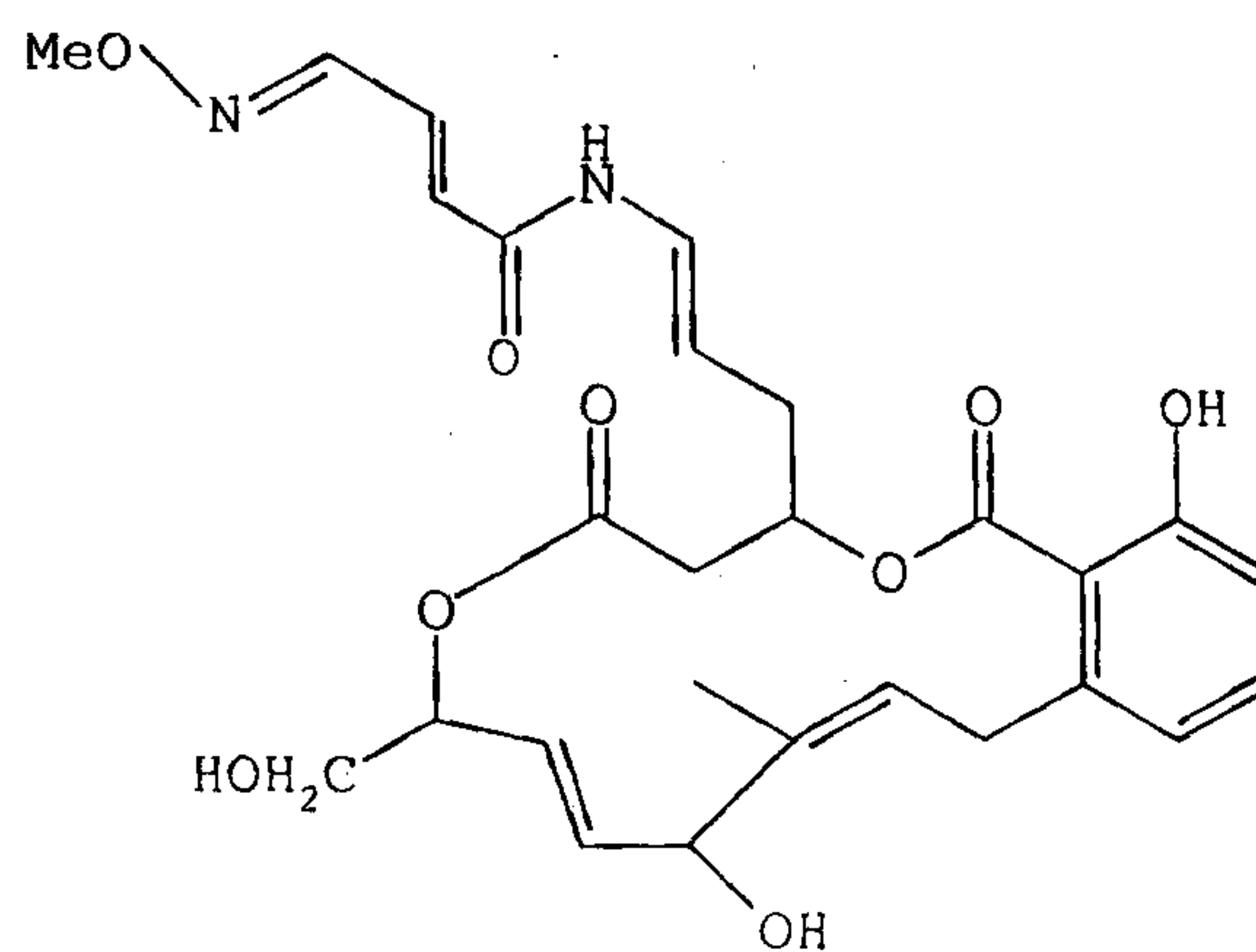
Lobatamide F;
