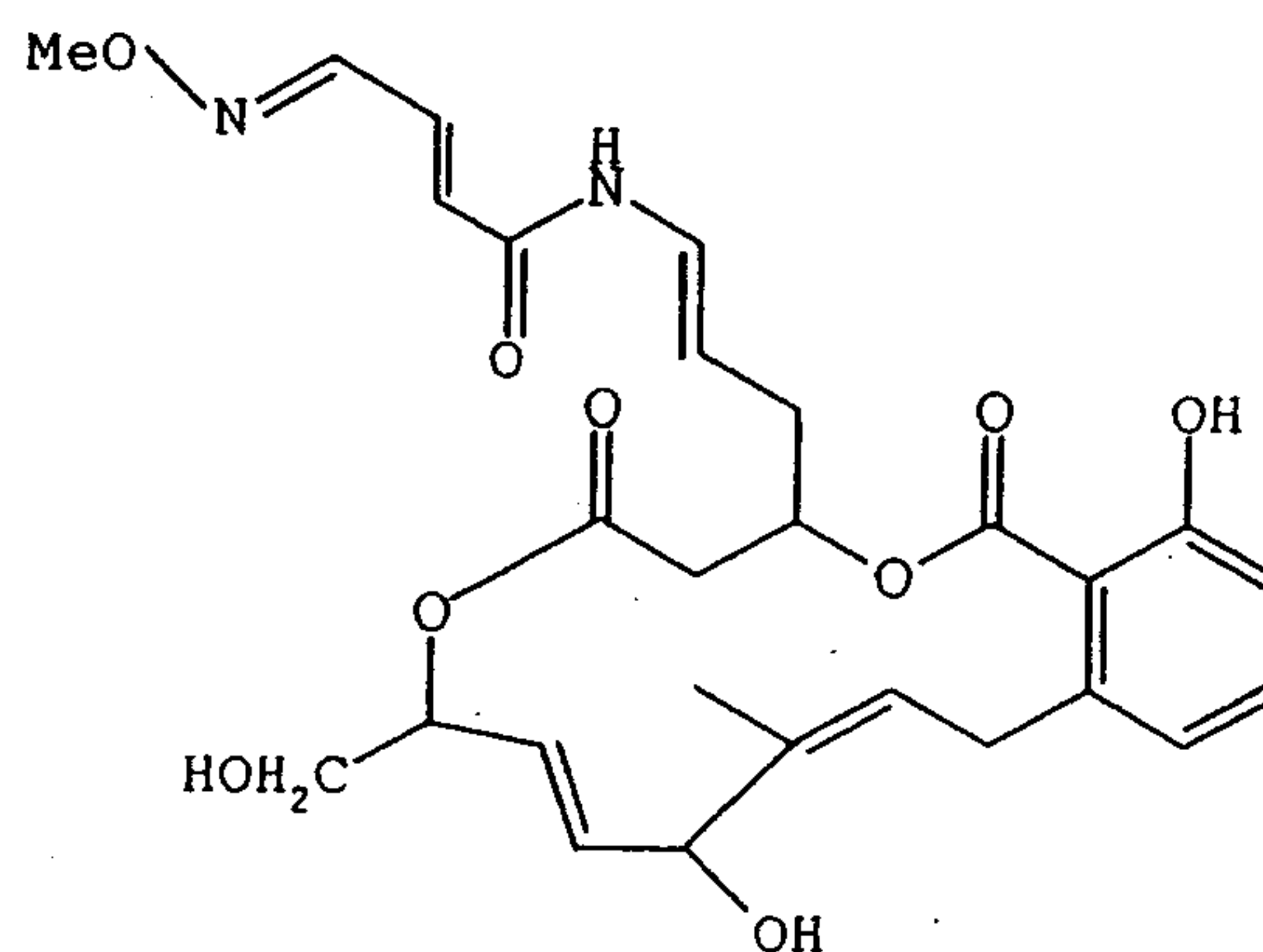
Lobatamide F;
