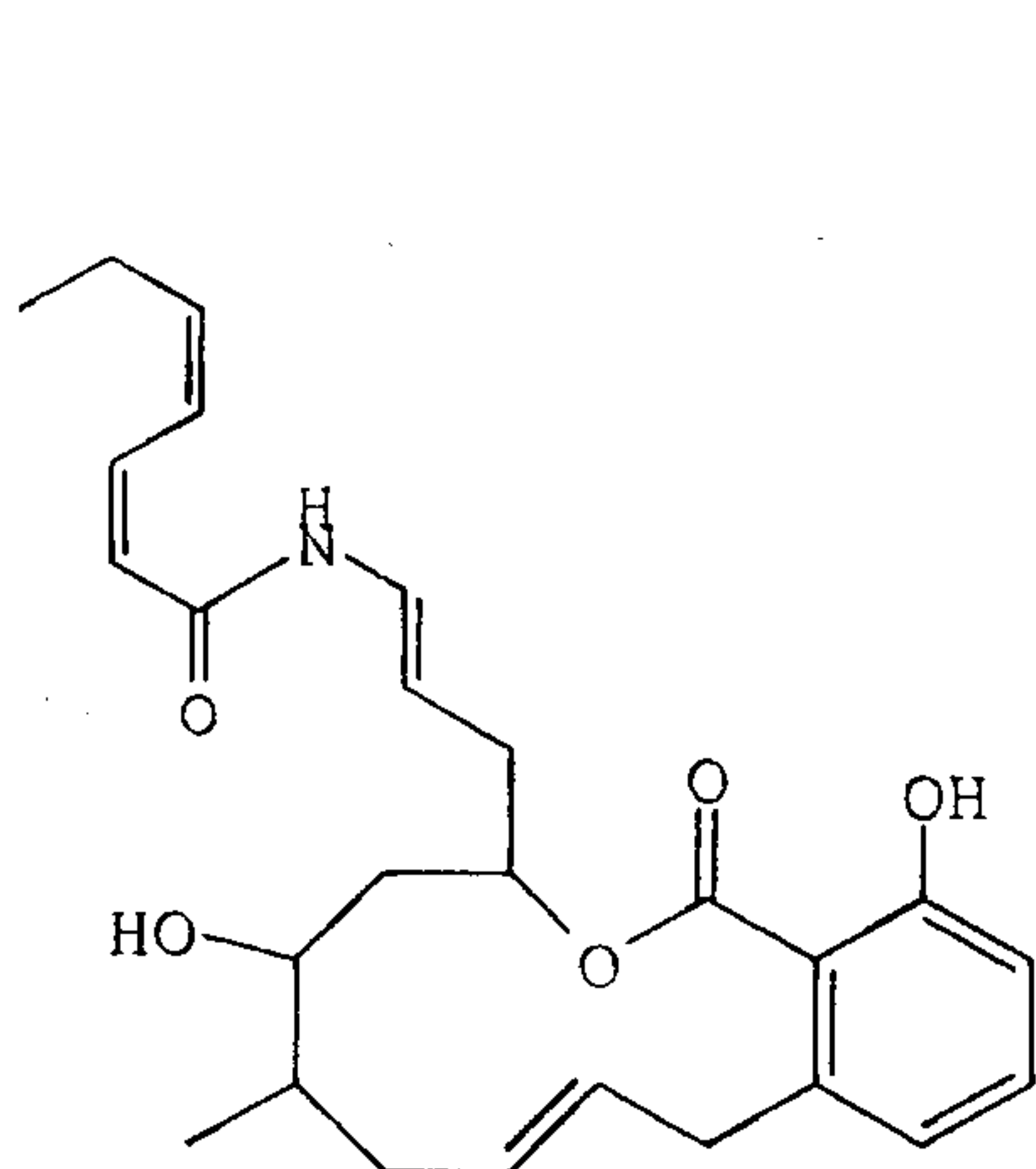
Salicylihalamide A,
