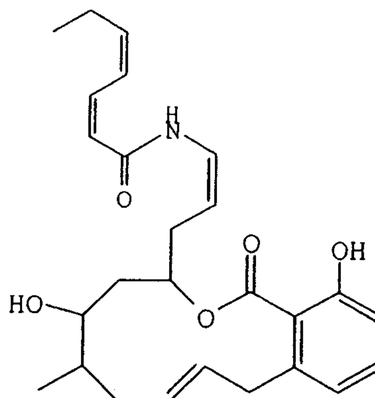
Salicylihalamide B,
