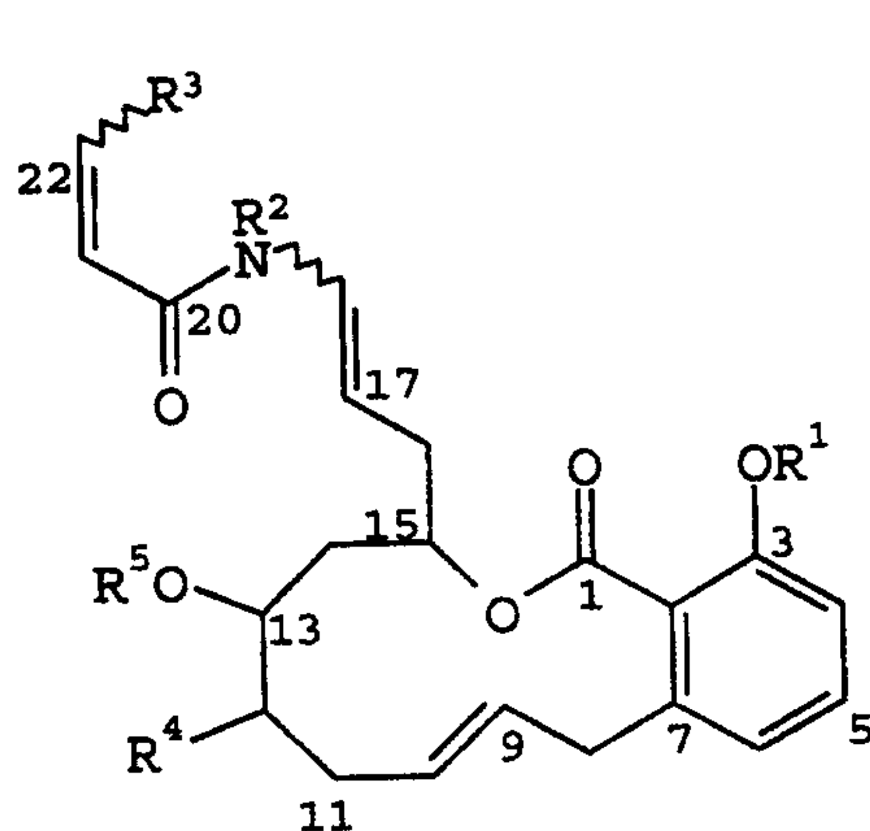
(IA)
