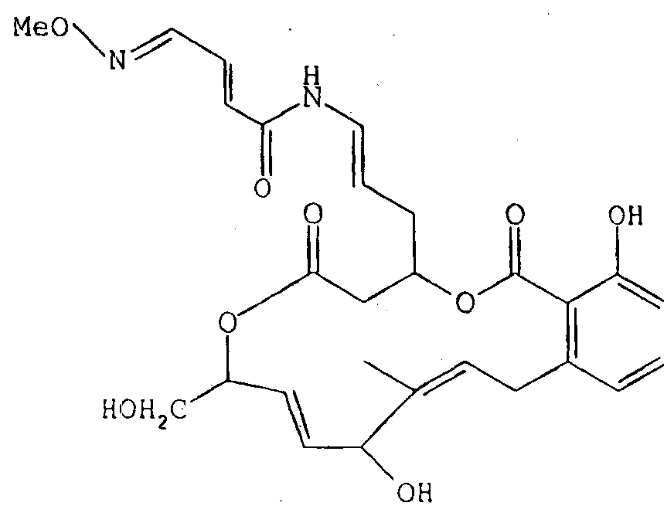
Lobatamide F;
