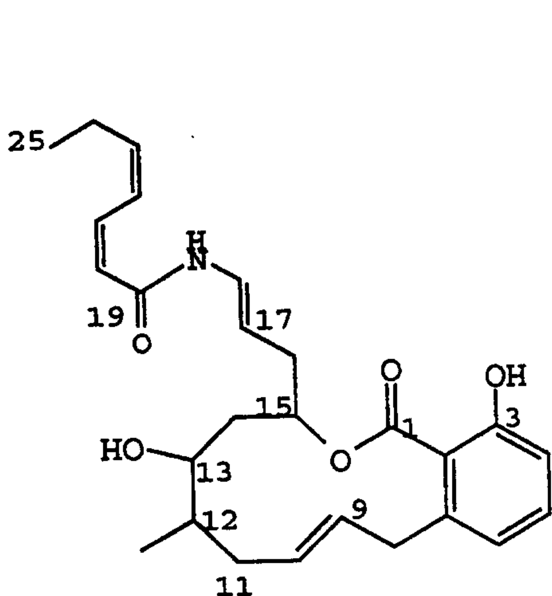
Salicylihalamide A;
