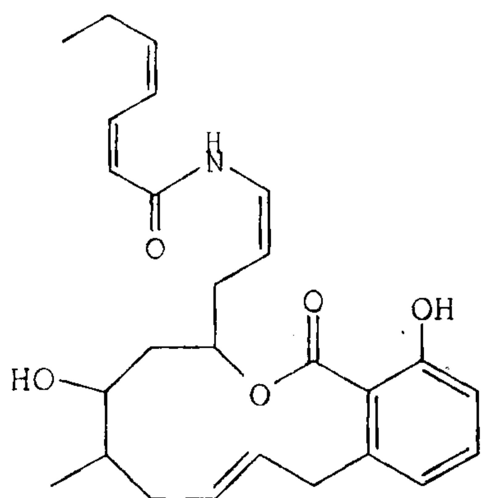
Salicylihalamide B,
