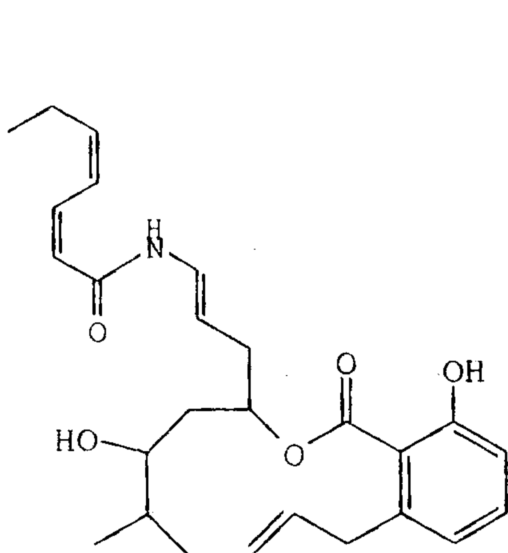
Salicylihalamide A,
