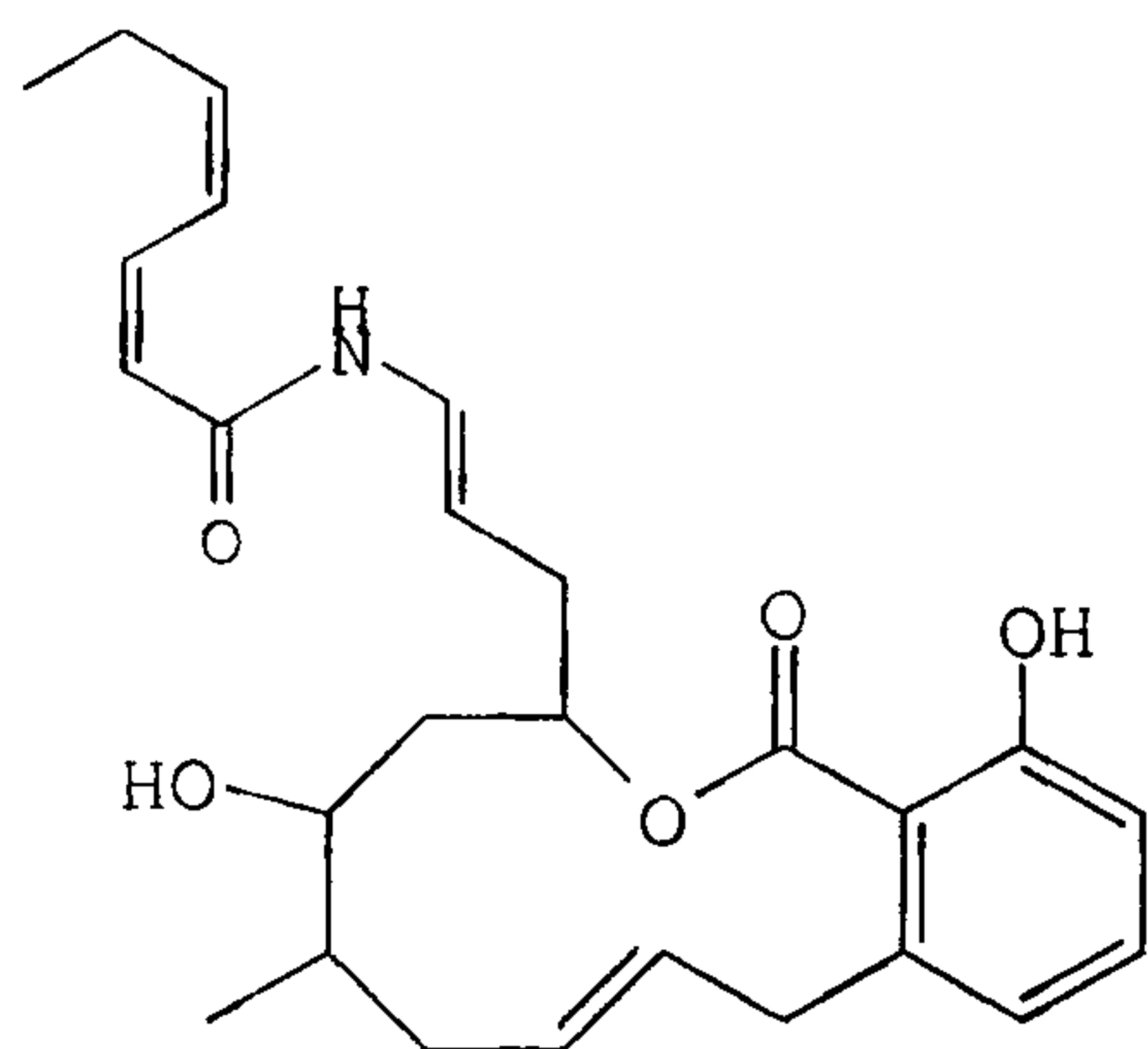
Salicylihalamide A,
