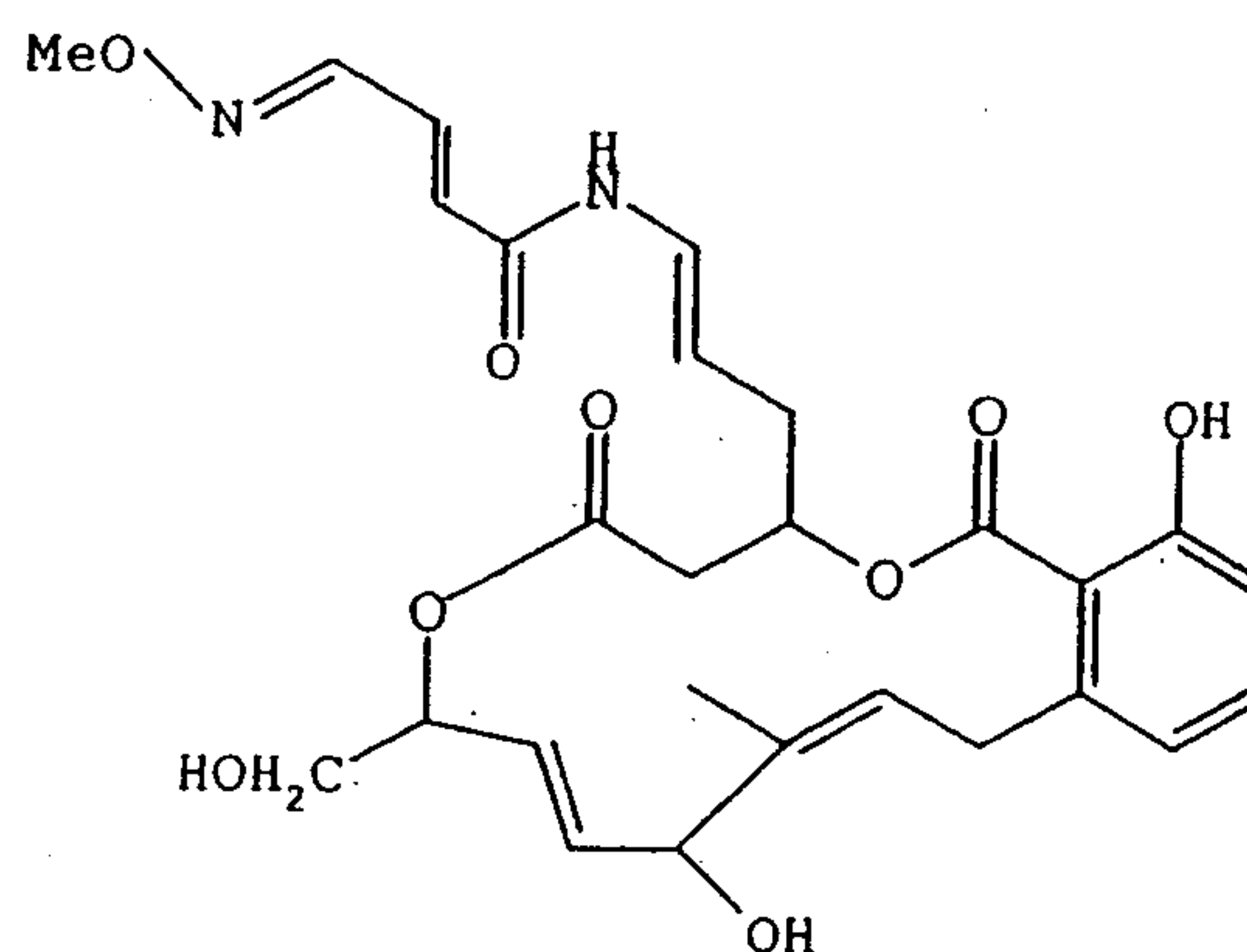
Lobatamide F;
