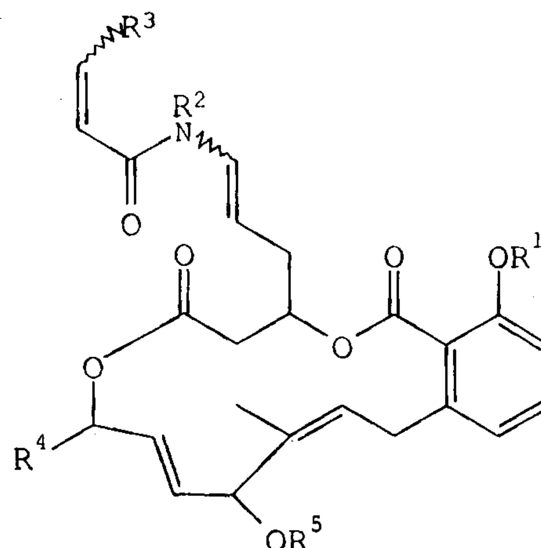
(IB),
