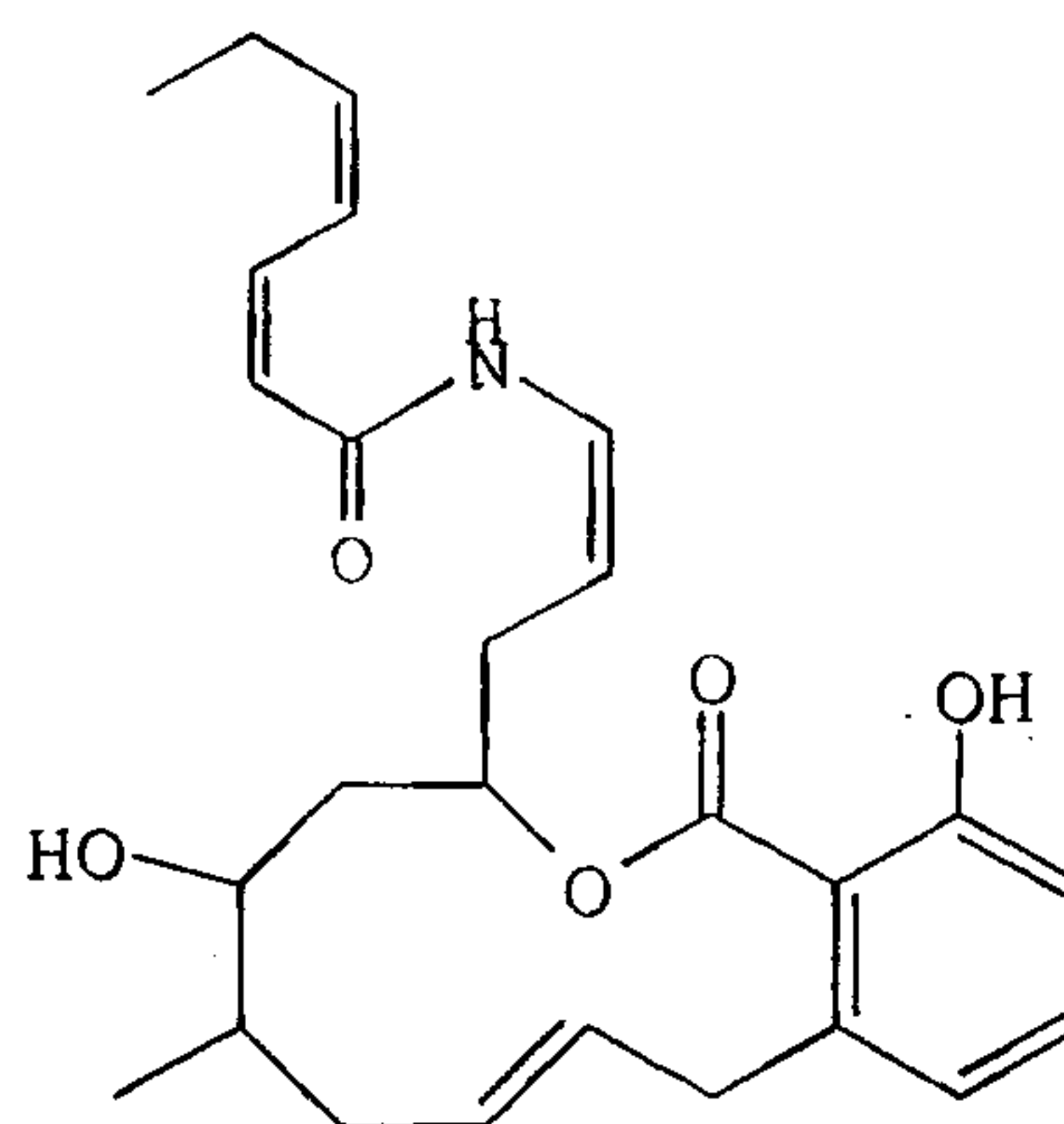
Salicylihalamide B,
