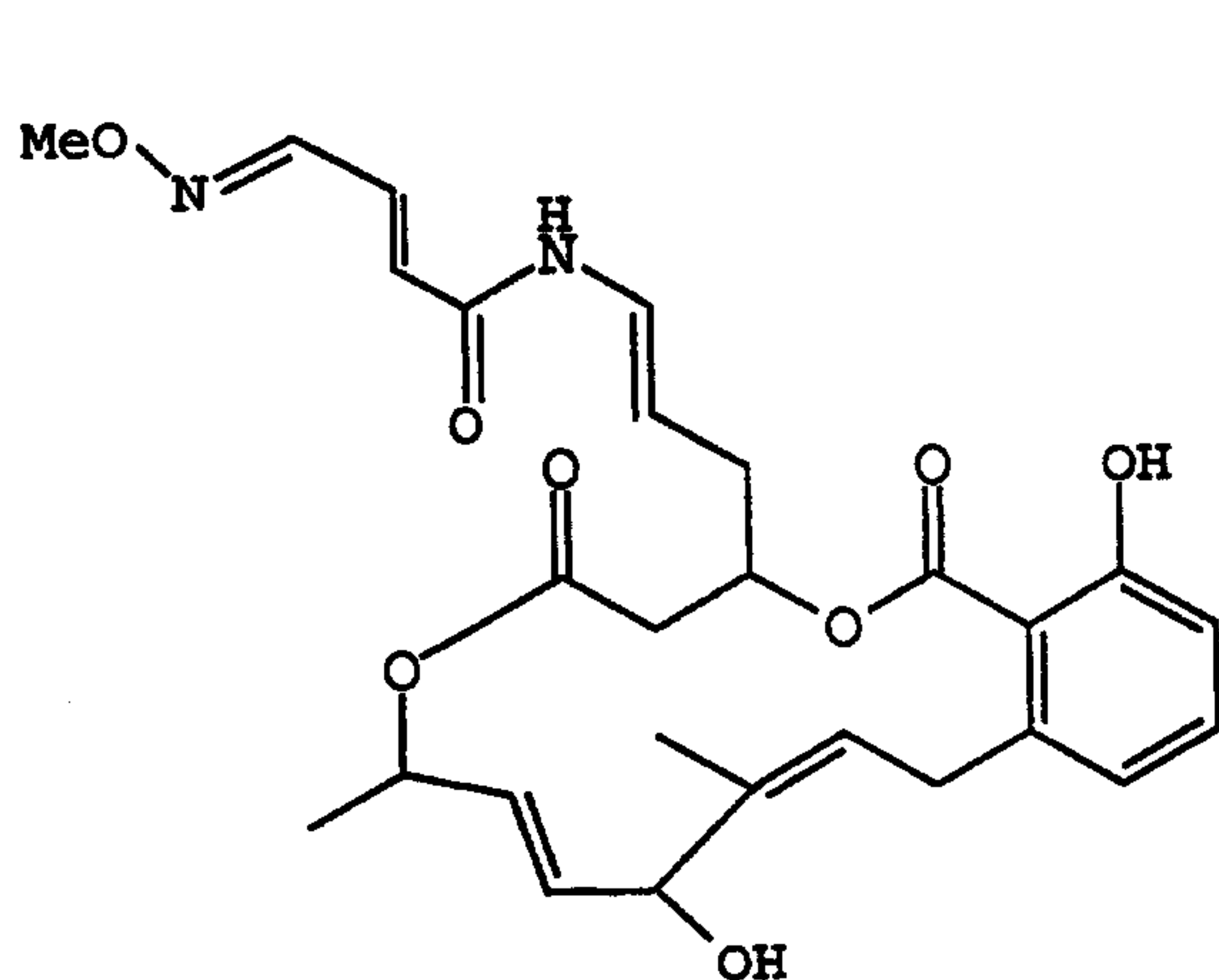
Salicylihalamide B;
