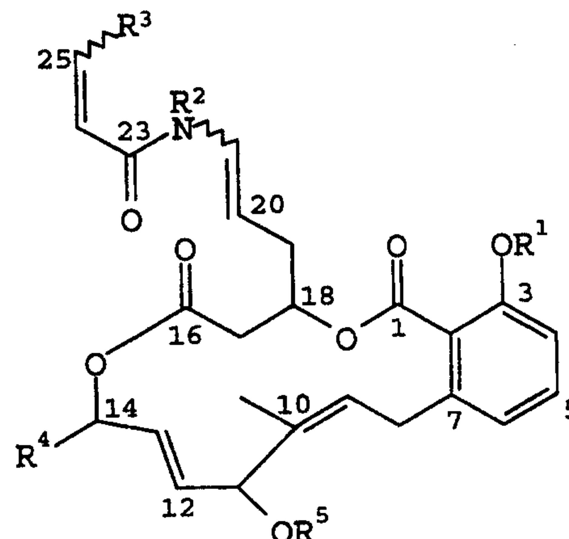
(IB),
