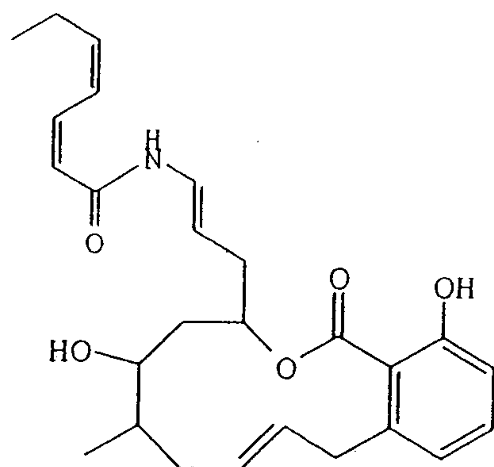
Salicylihalamide A,
