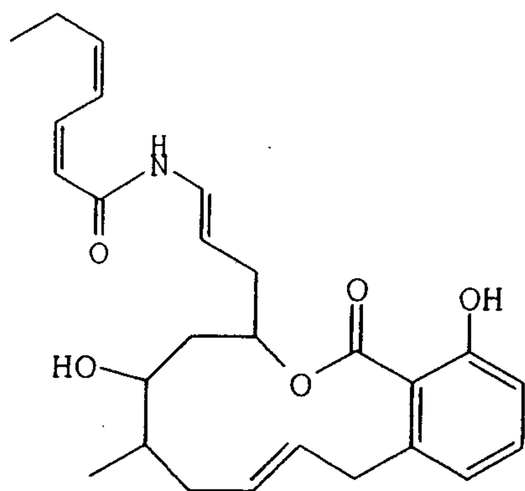
Salicylihalamide A,
