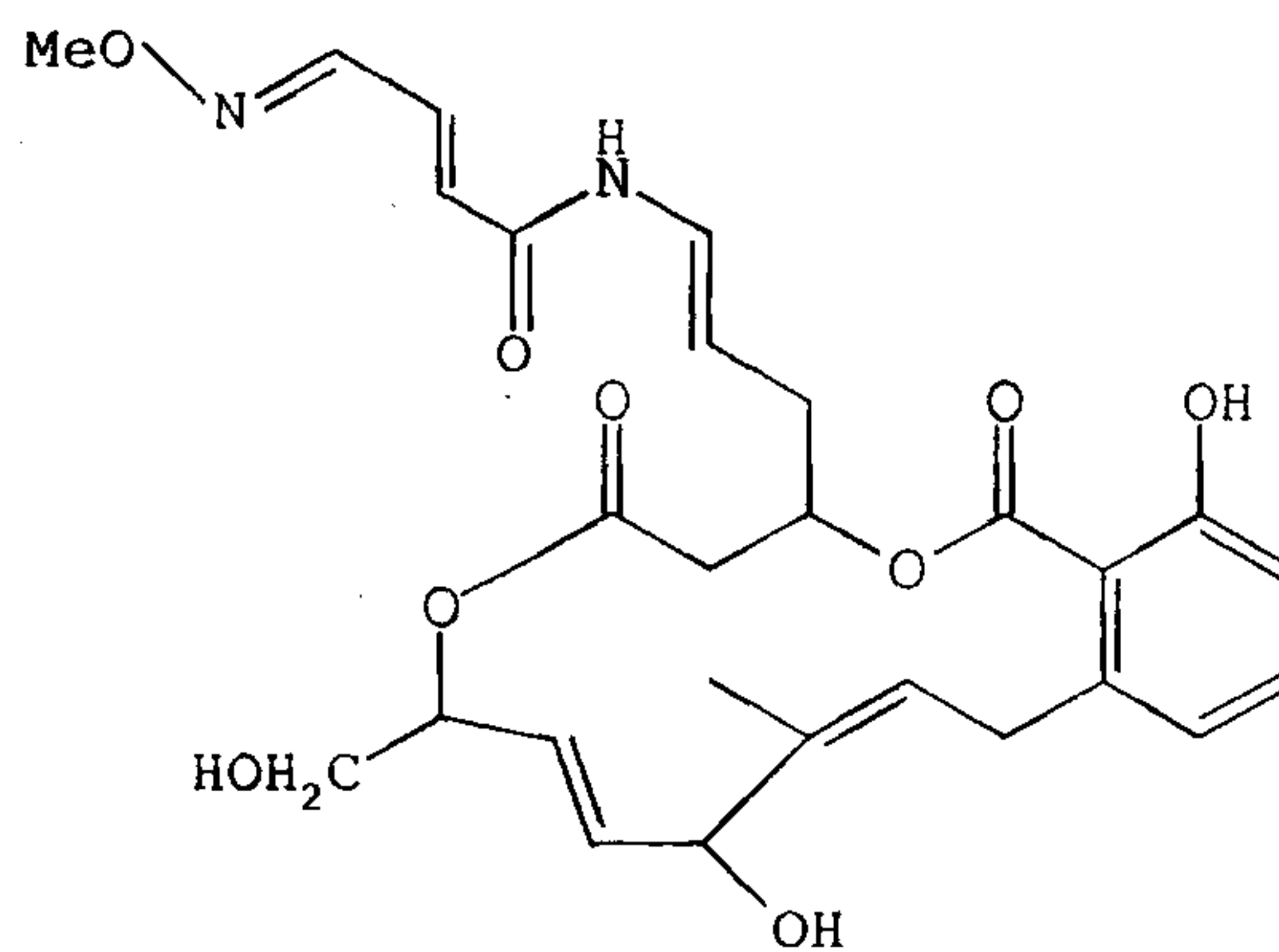
Lobatamide F;
