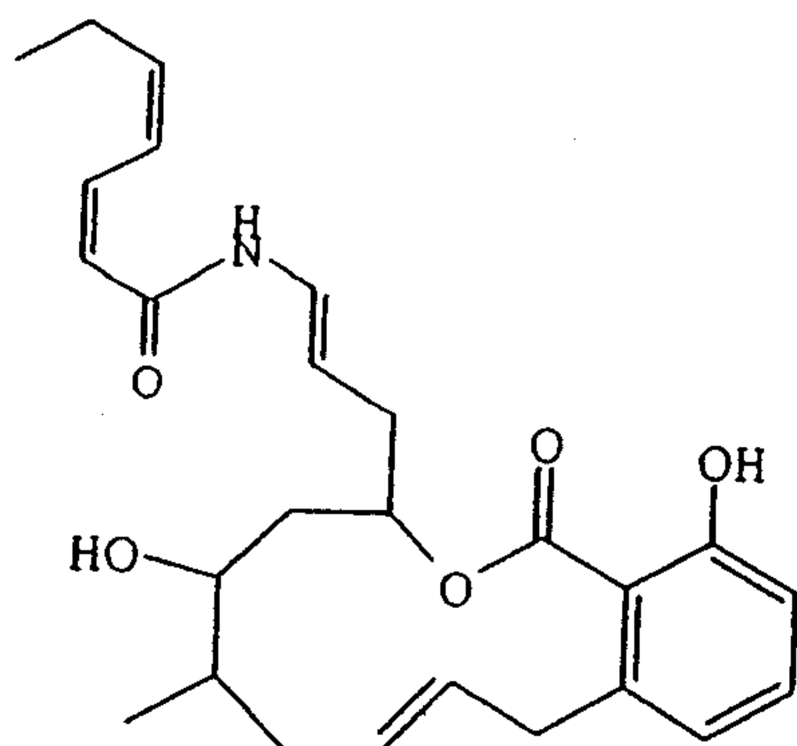
Salicylihalamide A,
