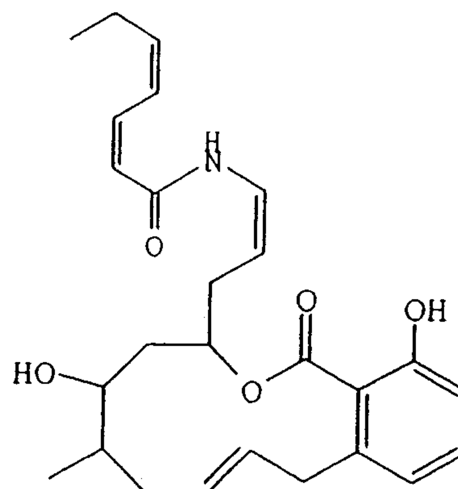
Salicylihalamide B,
