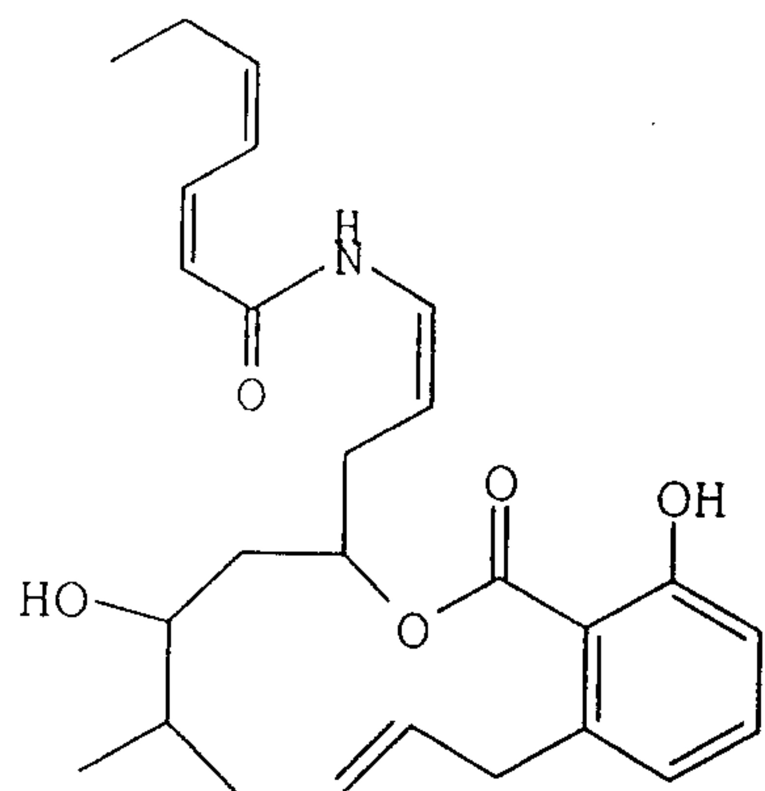
Salicylihalamide B,
