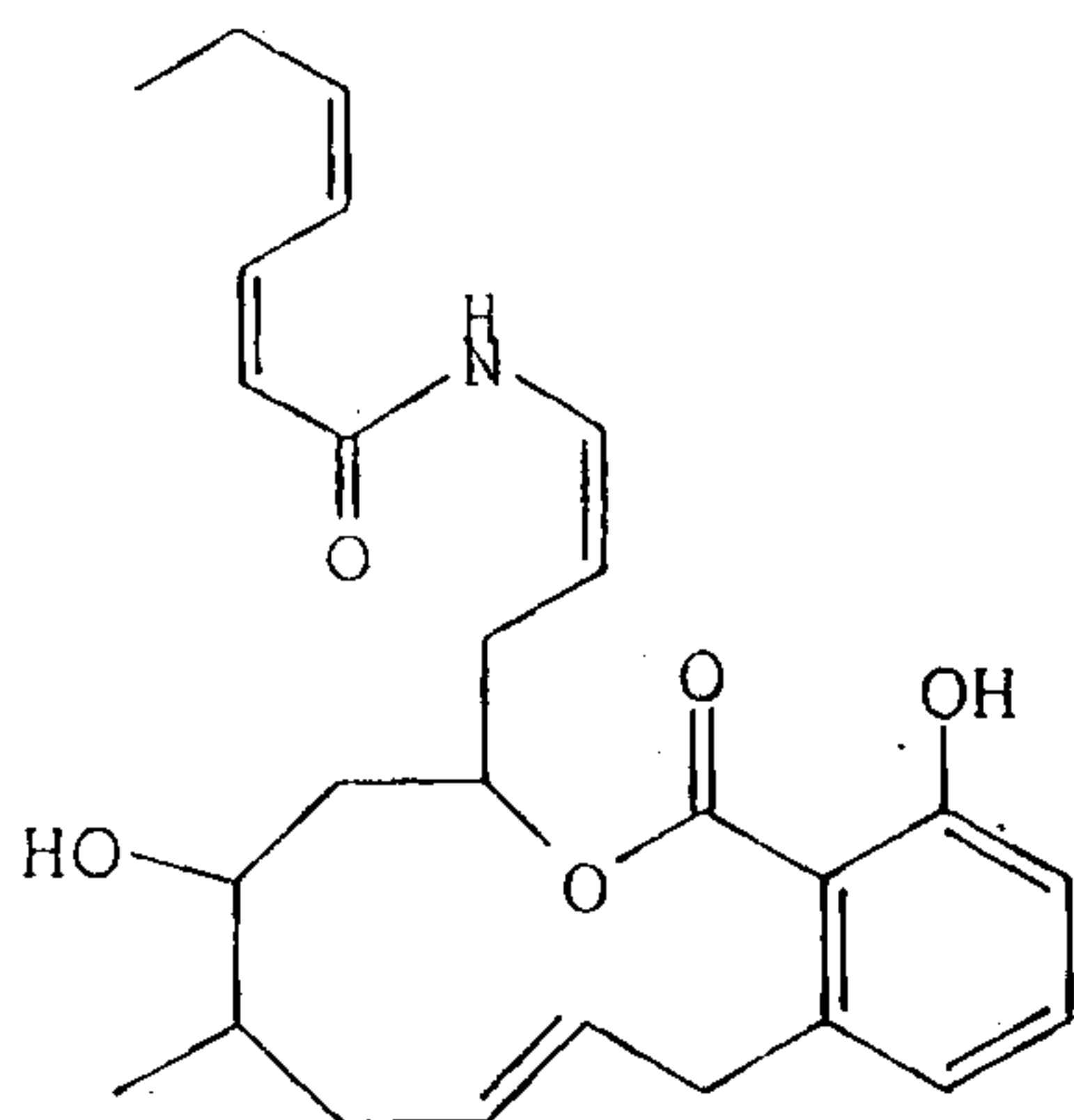
Salicylihalamide B,
