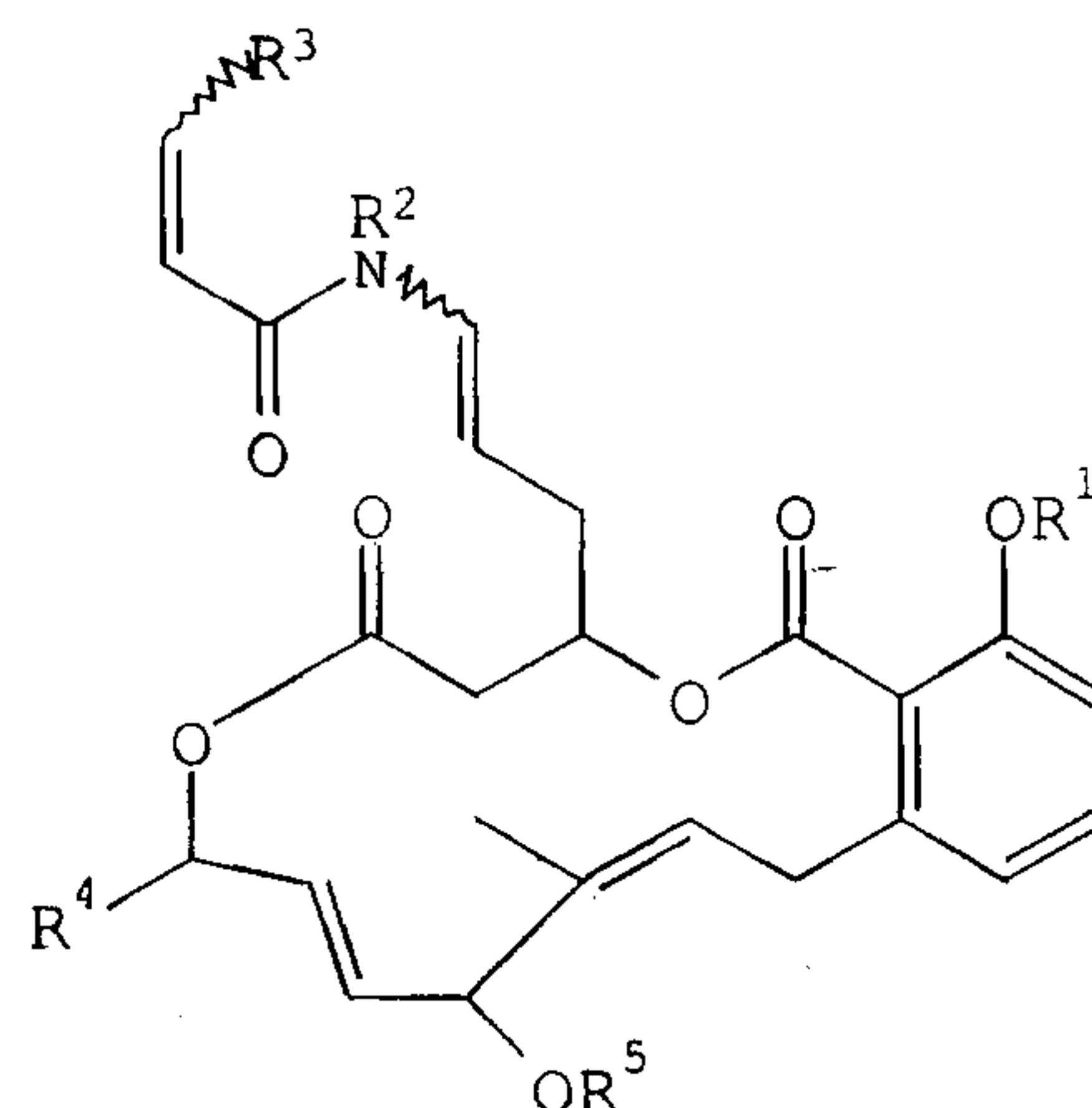
(IB),
