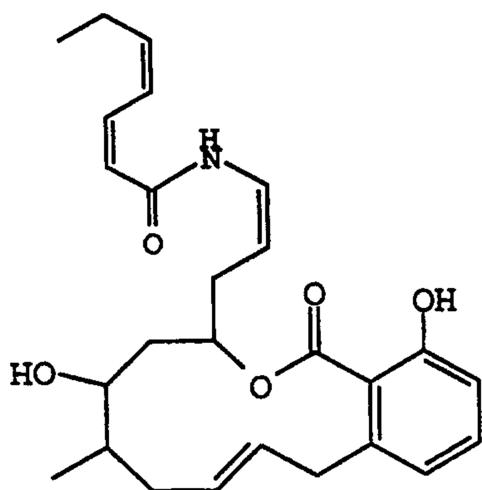
Salicylihalamide B;
