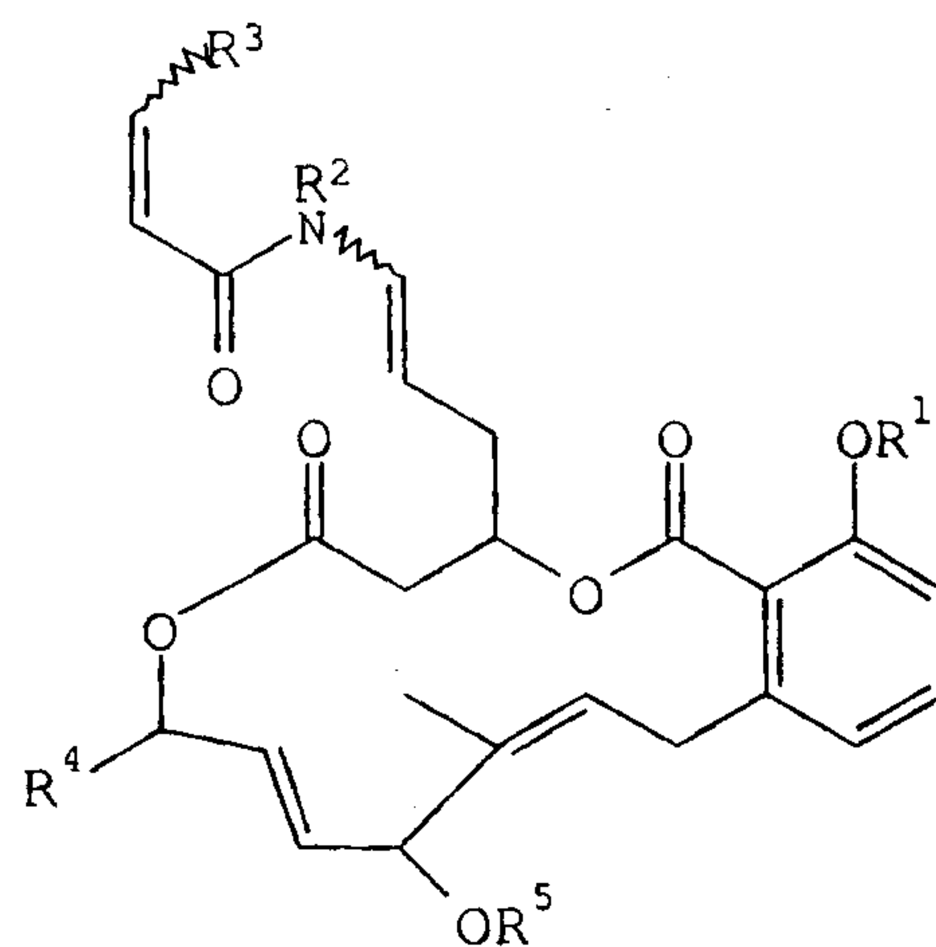
(IB),
