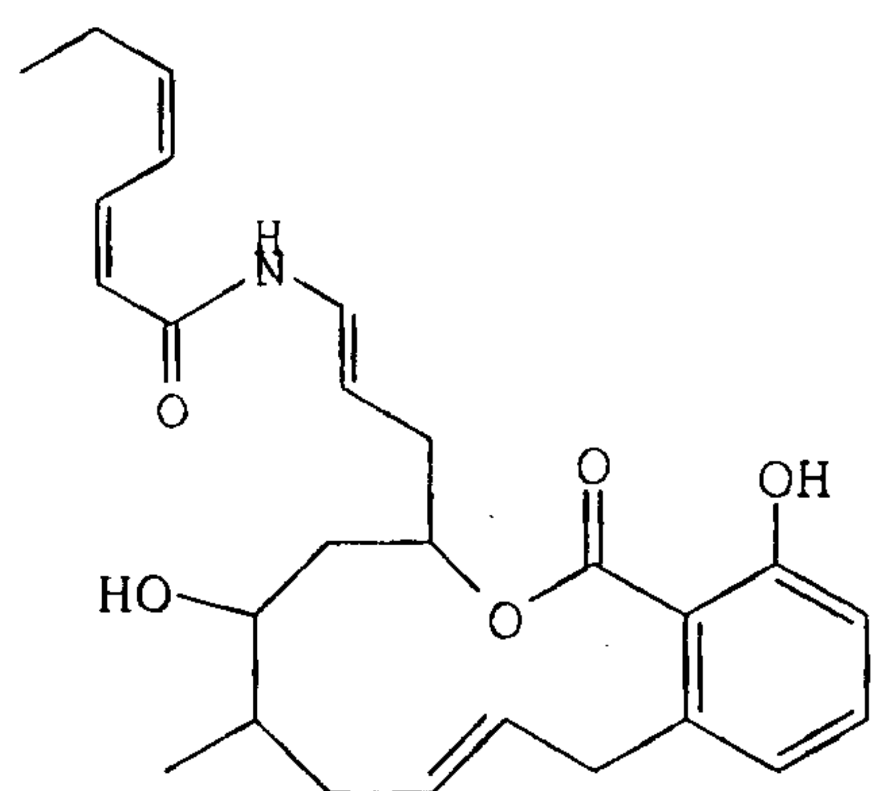
Salicylihalamide A
