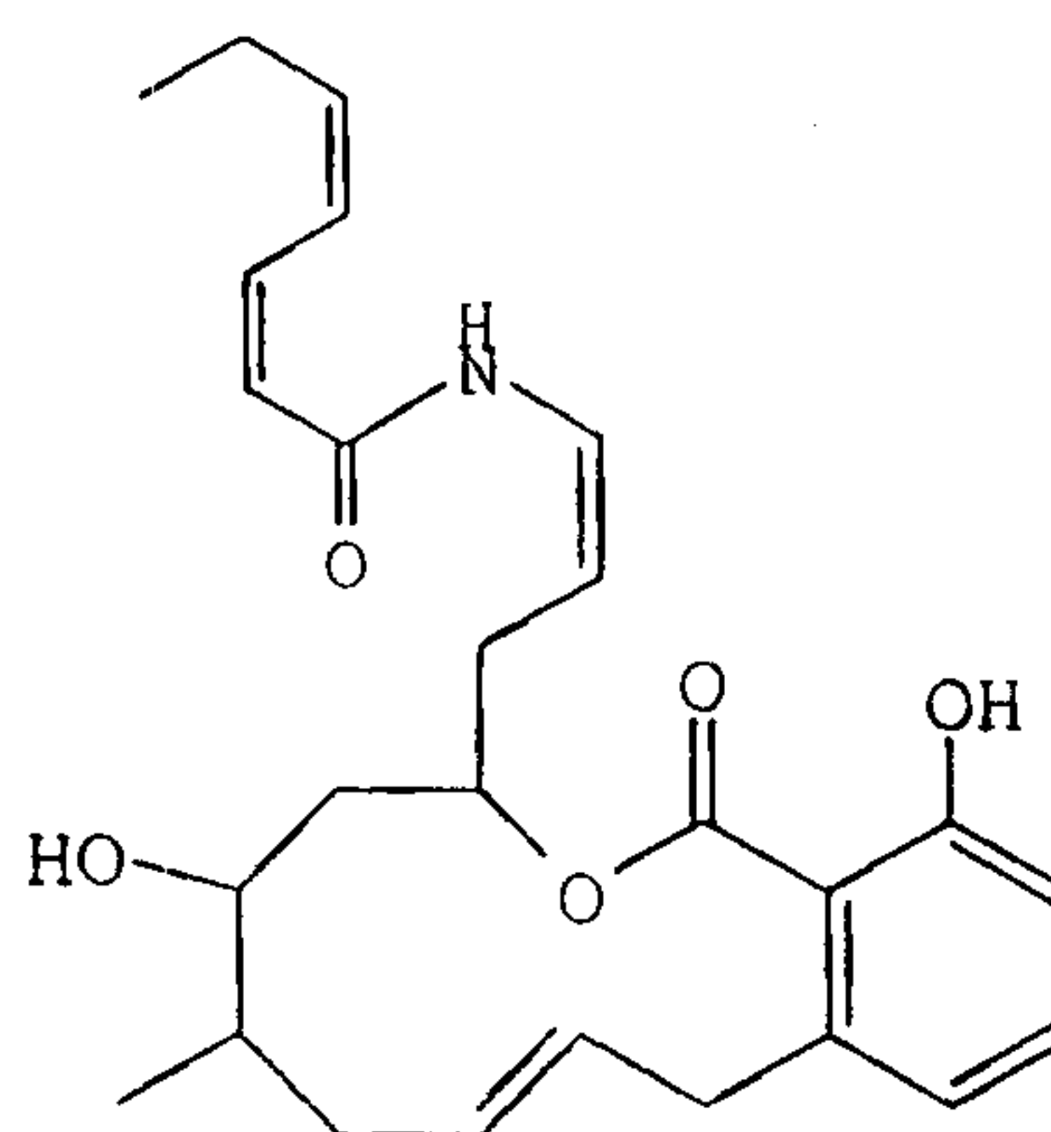
Salicylihalamide B;
