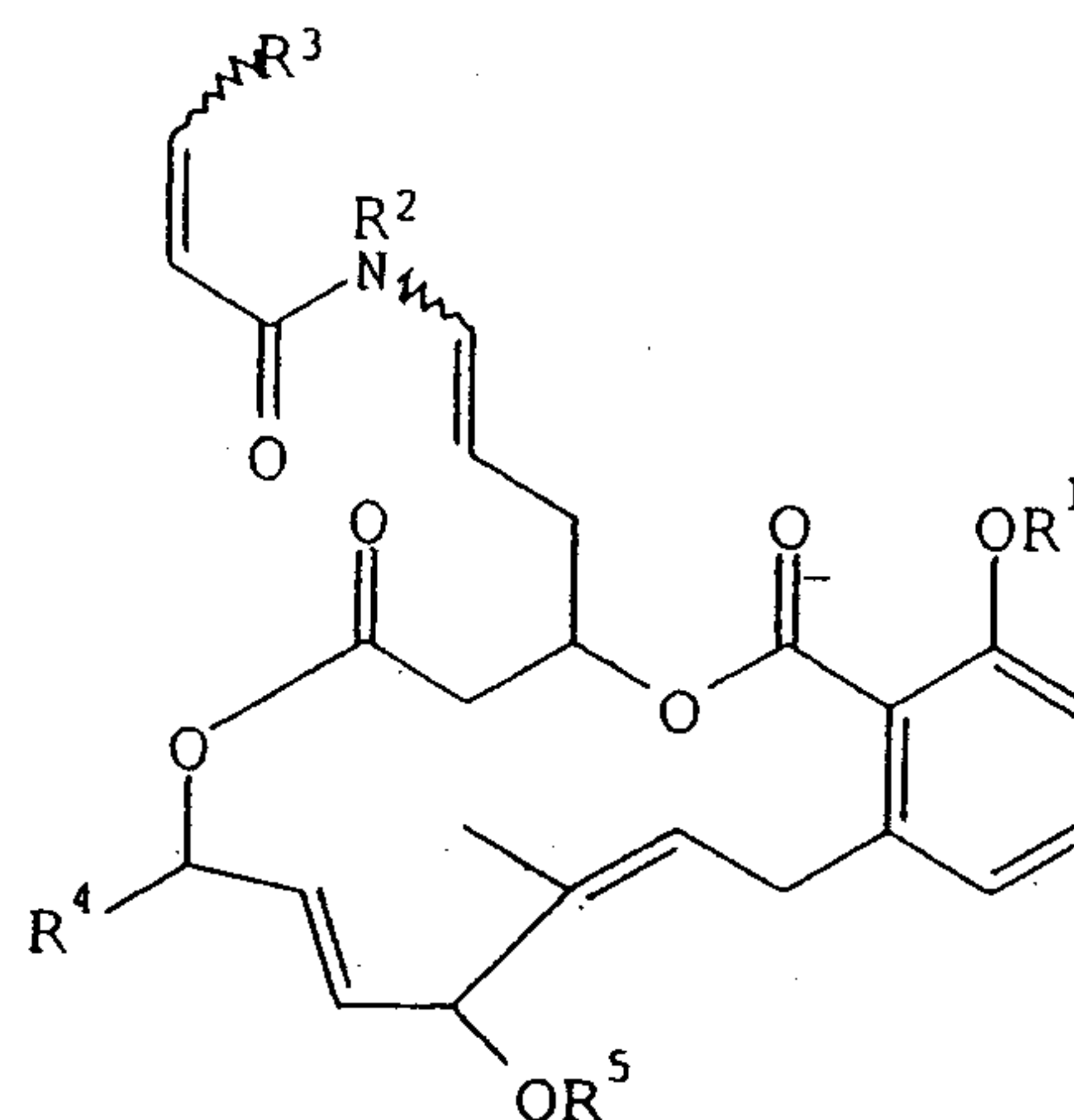
(IB),
