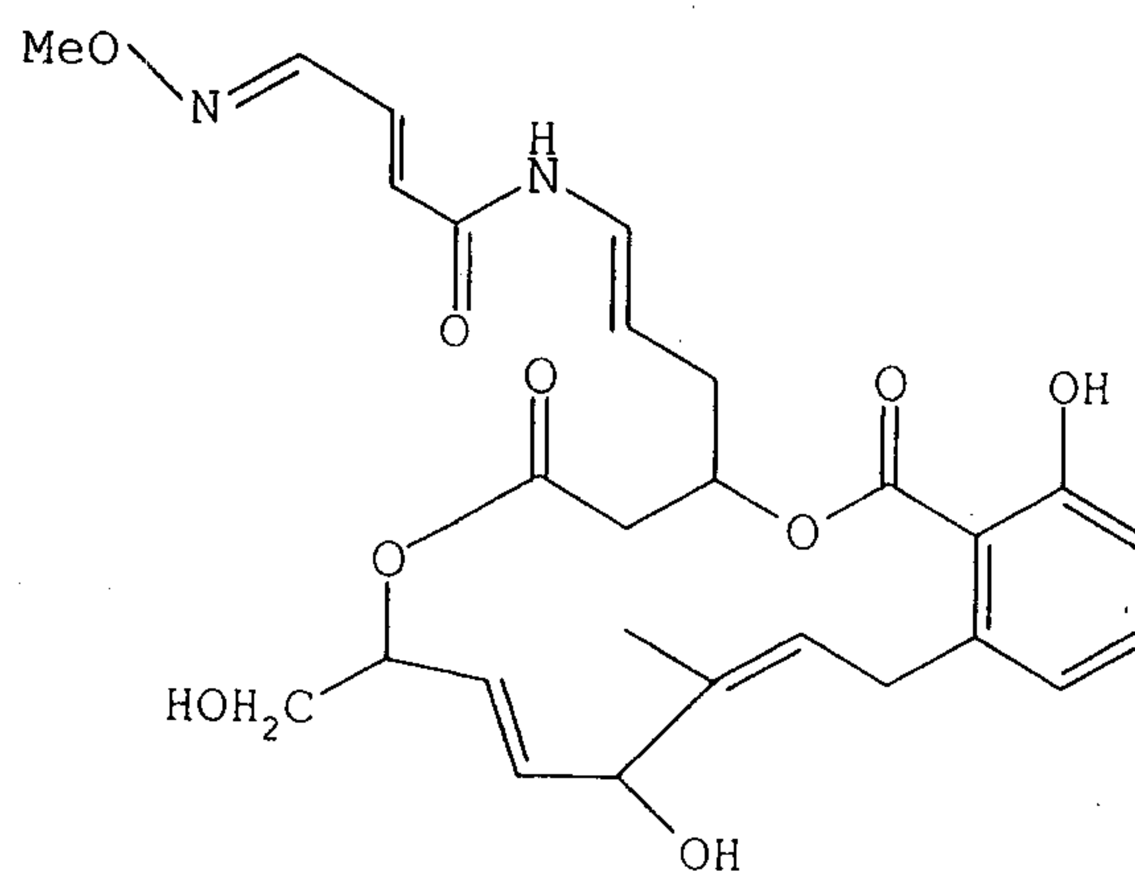
Lobatamide F;
