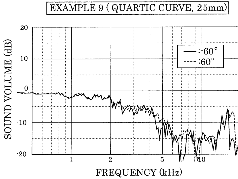
FIG. 26A
