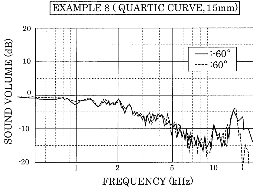
FIG. 23A
