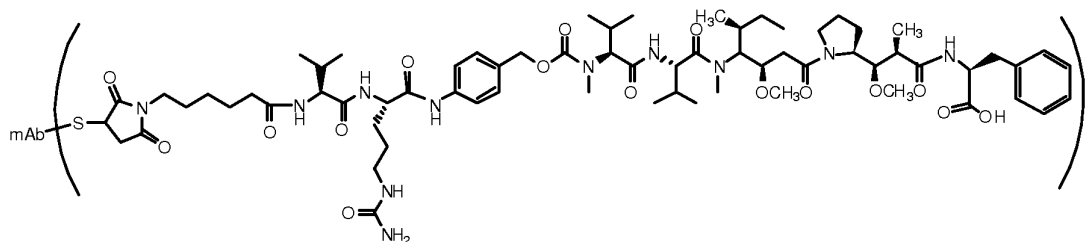
L-mc-vc-MMAF
