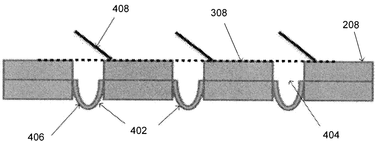
FIG. 4C
