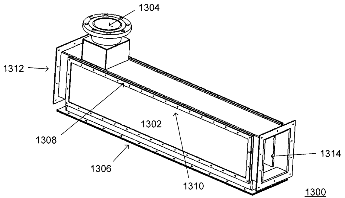
FIG. 13A
