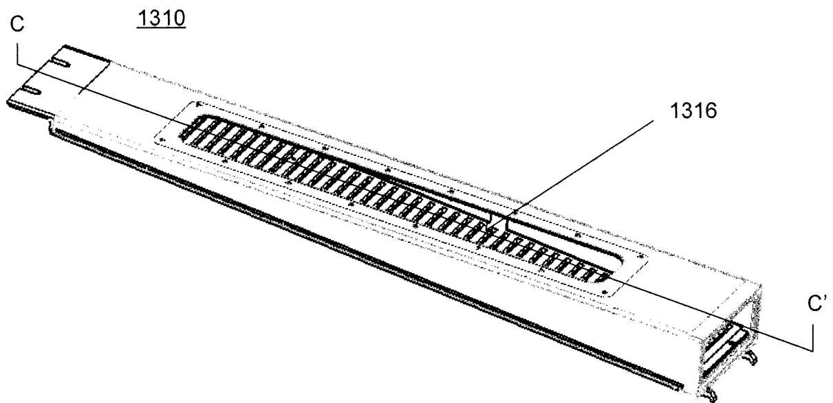
FIG. 13B
